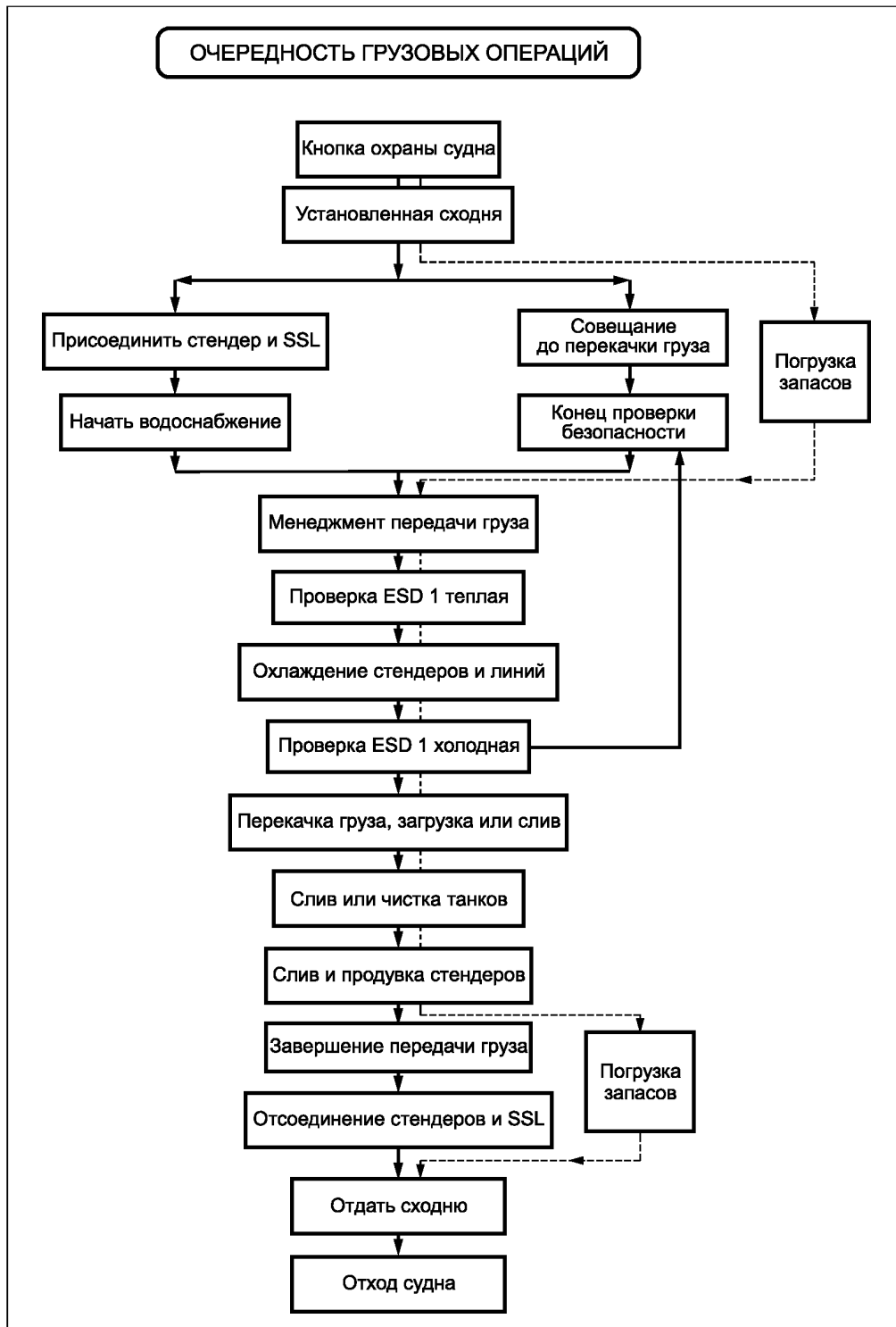
Рисунок В.1 — Типовая блок-схема грузовых операций
