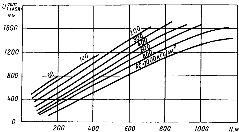
Рис. 28. Смещения пород в зоне остаточного опорного давления при охране выработок бутовыми полосами и кострами
