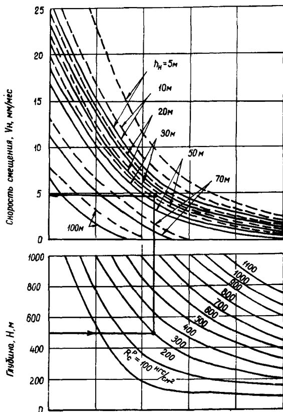
Рис. 65. Номограмма для определения скорости смещения пород в надрабатываемых полевых (сплошная кривая) и пластовых (пунктирная кривая) выработках
