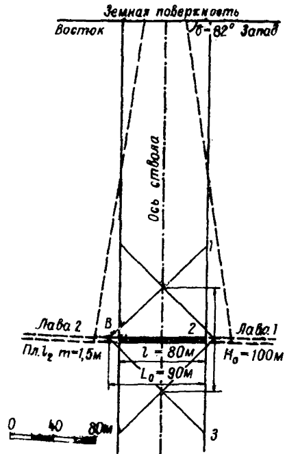
Рис. 52. Схема расчета деформаций ствола к примеру 4
