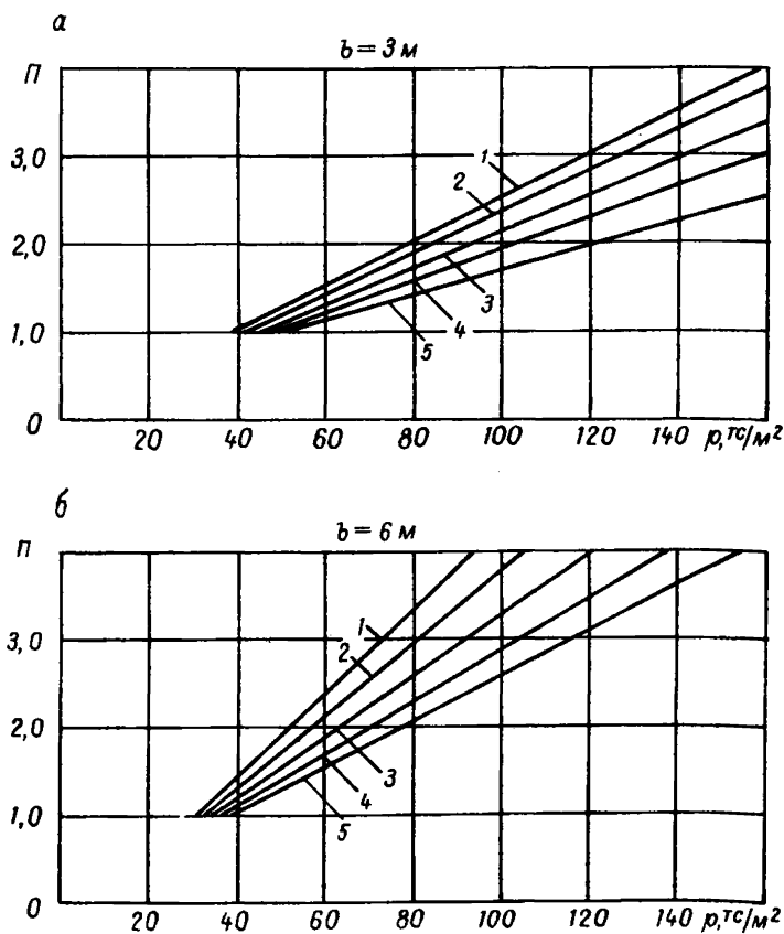
Рис. 13. Графики для выбора плотности установки двутавровых рам железобетонной крепи в однопутевой (а) и двухпутевой (б) выработках в зависимости от величины расчетной нагрузки на крепь и номера двутаврового профиля:
