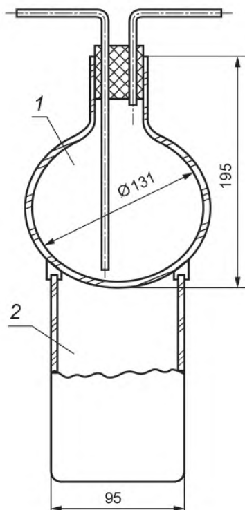
1 — круглодонная колба; 2 — высокий стеклянный стакан
