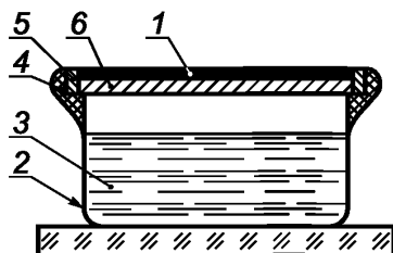
1 — испытуемый слой СФТК; 2 — стеклянная чашка; 3 — дистиллированная вода; 4 — герметизирующая мастика; 5 — слой парафина; 6 — основание (утоплитель)
