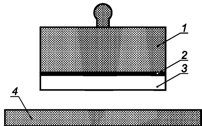
а) АТС-1 — отрыв по границе «образец — основание»
