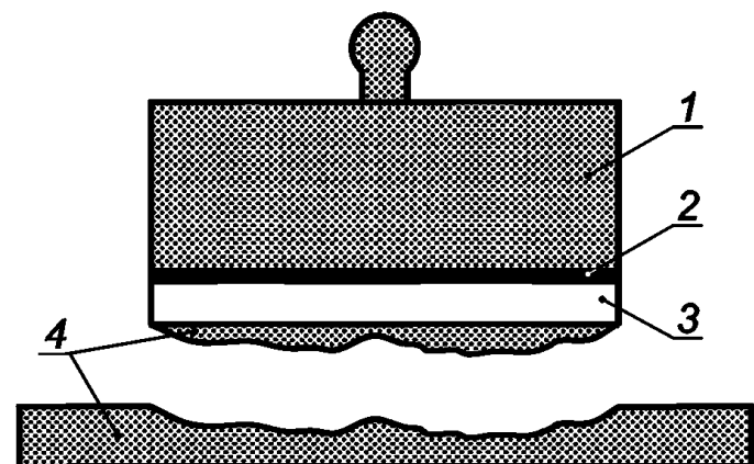
в) АТС-3 — отрыв по телу основания
