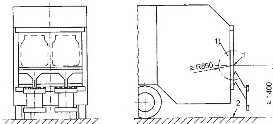
Закрытая система подъема
