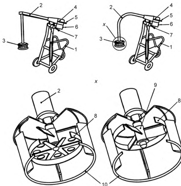
1 – передвижная тележка; 2 – консоль; 3 – рабочая головка; 4 – двигатель; 5 – рукоятка управления; 6 – устройство пуск/останов; 7 – рукоятка фиксации; 8 – статор; 9 – инструмент; 10 – защитное устройство рабочей головки
