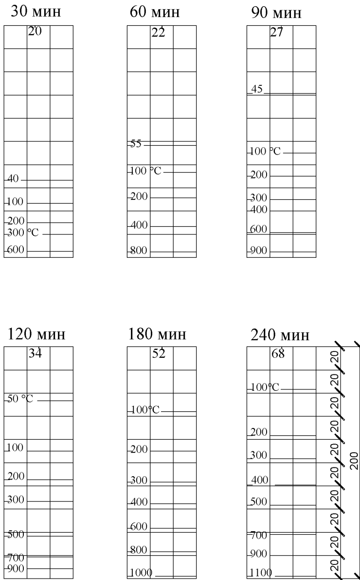
Рисунок И.12 - Плита из тяжелого бетона толщиной 200 мм при нагреве с одной стороны
