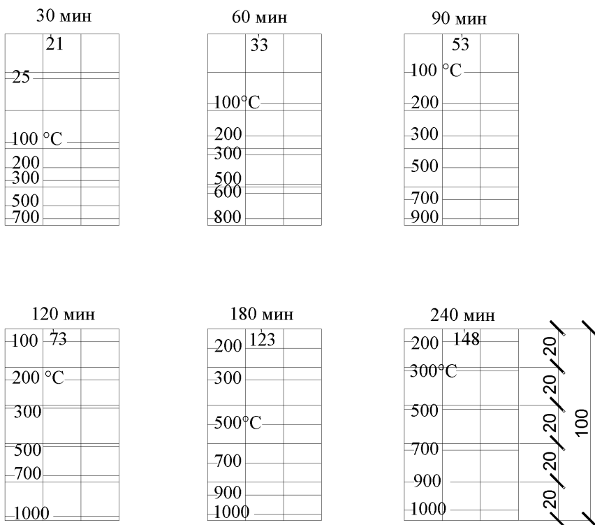
Рисунок И.14 - Плита из легкого бетона толщиной 100 мм при нагреве с одной стороны
