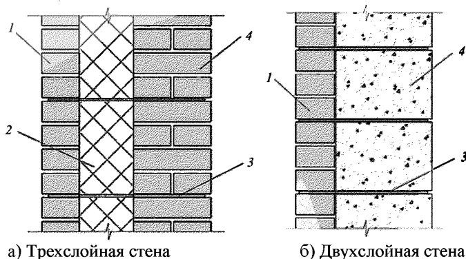
Рисунок 8.1 – Стены с гибкими связями между слоями
