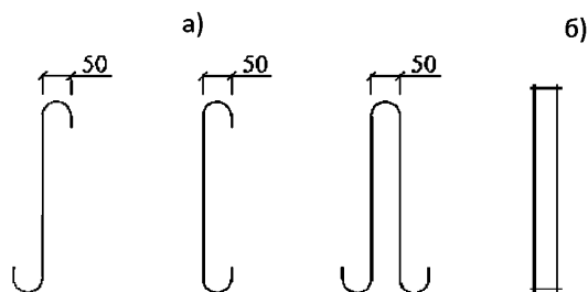
Рисунок 7.1 – Одиночные гибкие связи
