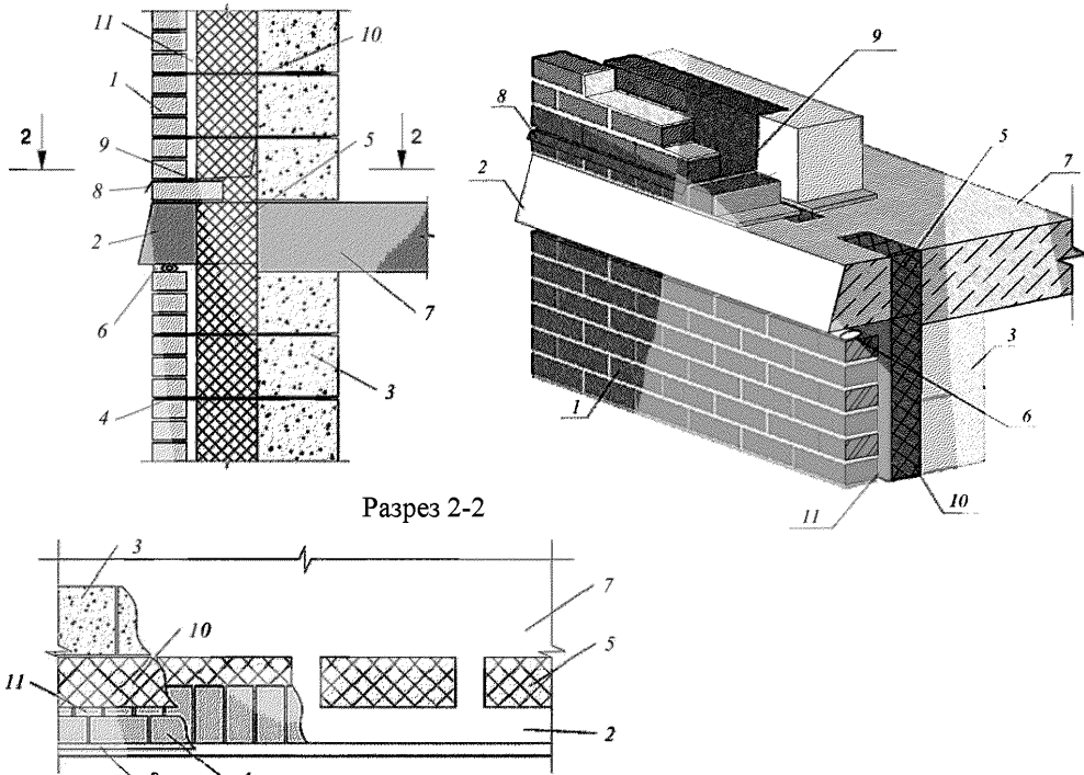
Рисунок 8.4 – Наружные двухслойные стены с лицевым слоем, опирающимся на плиту перекрытия
