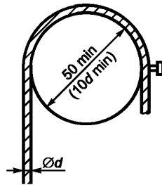
Рисунок 1 — Устройство для удерживания испытуемого образца корда
