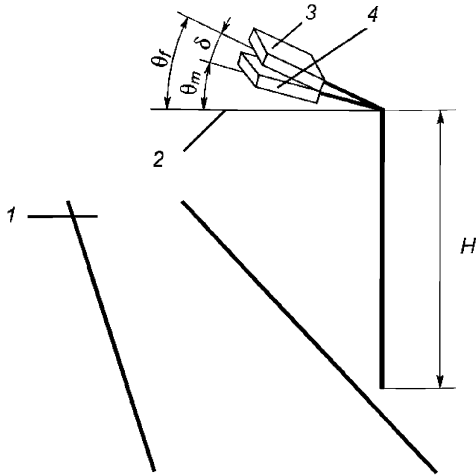
1 – дорога; 2 – горизонталь; 3 – ОП в положении при использовании (\theta_r) ; 4 – ОП в положении при измерении \theta_m
