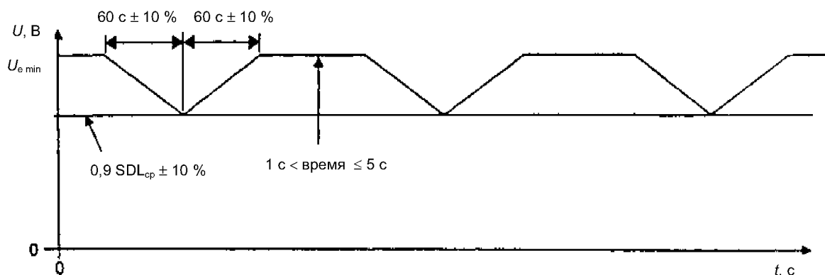
Рисунок 10 – Испытание на медленное изменение напряжения питания
