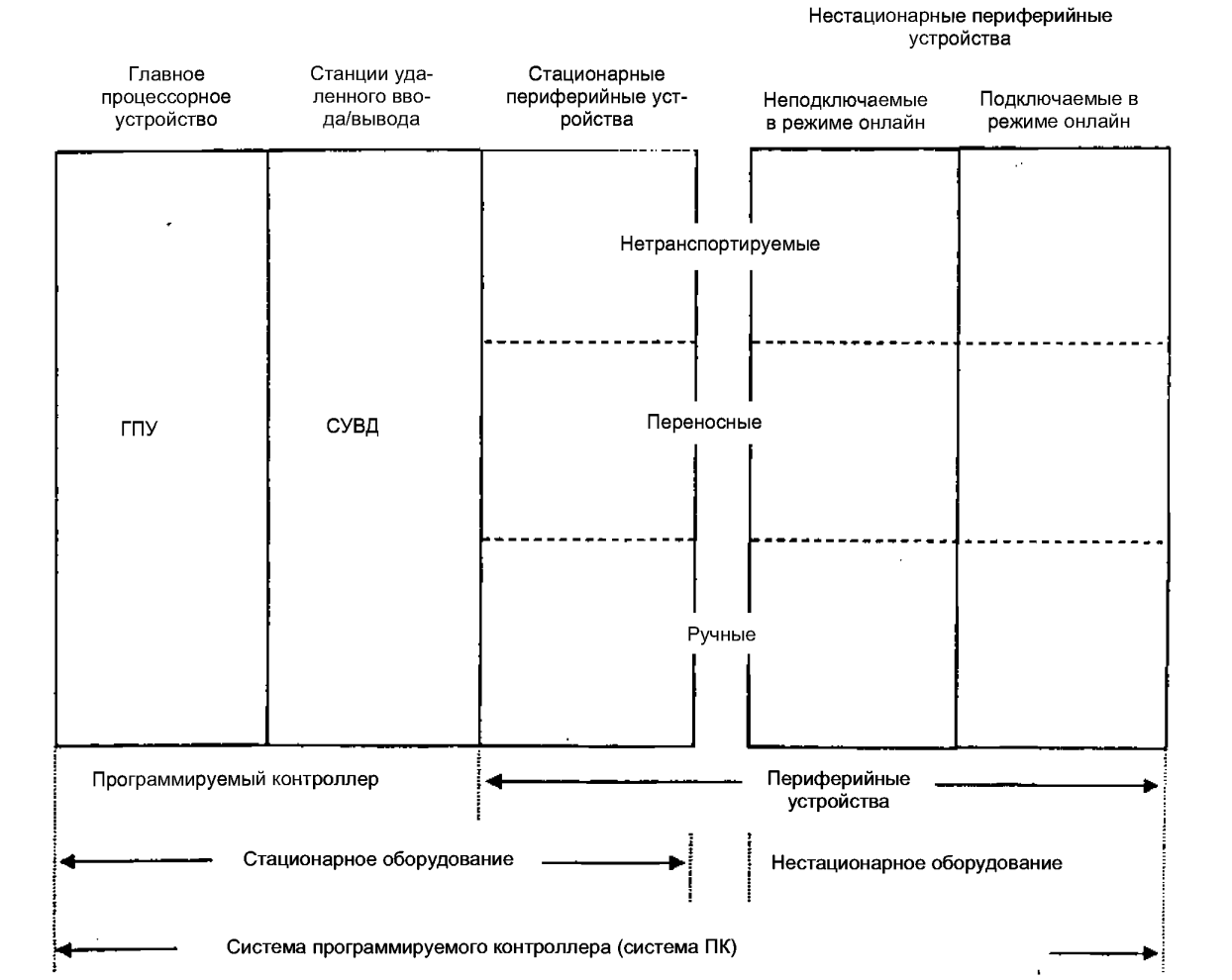
Рисунок А.1 – Система программируемого контроллера (система ПК)
