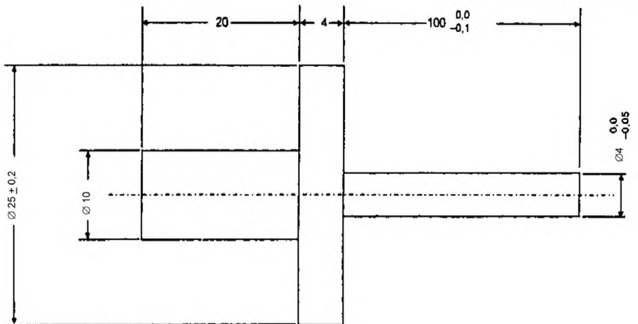
Рисунок С.3 – Испытательный штифт 100 × 4 мм
