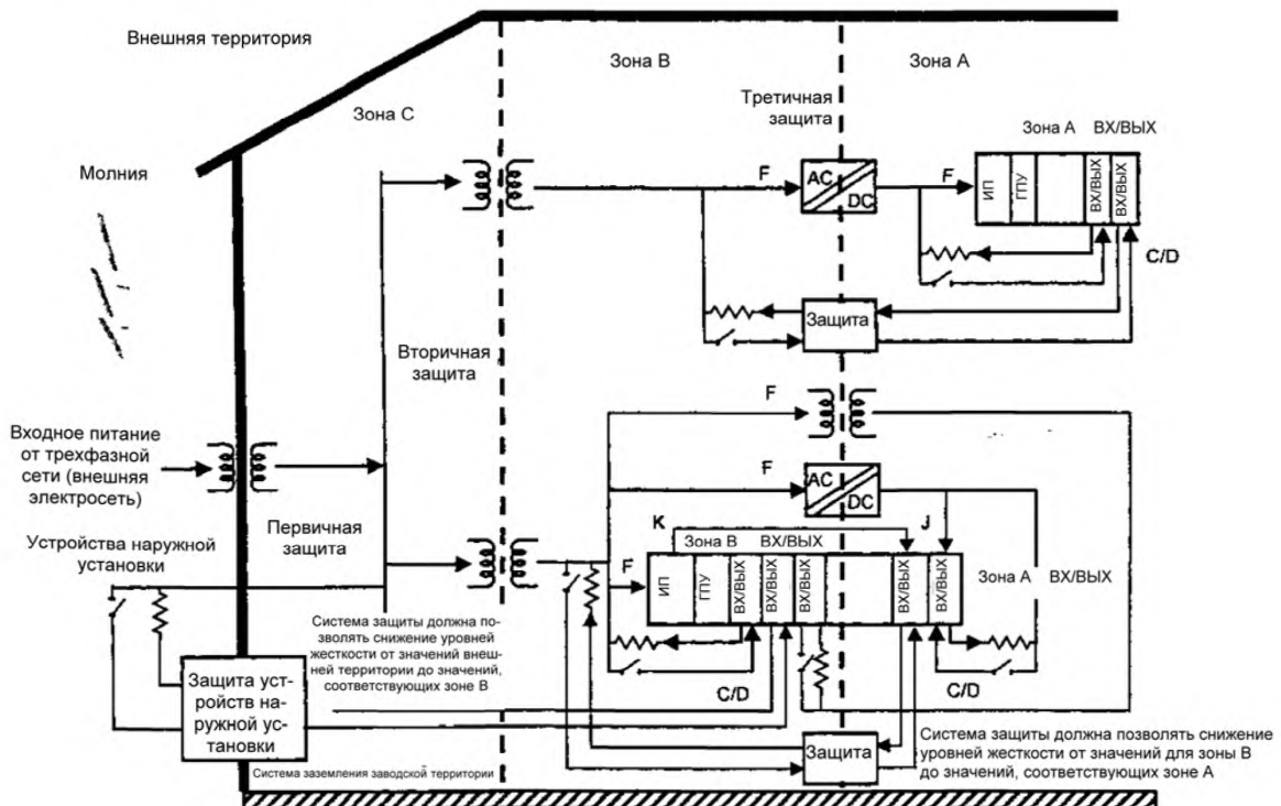
Рисунок 11 – Зоны устойчивости к электромагнитным помехам
