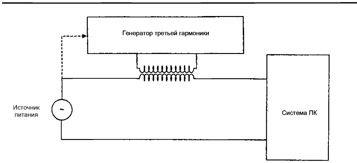
Рисунок 7 – Испытание на устойчивость к напряжению третьей гармоники
