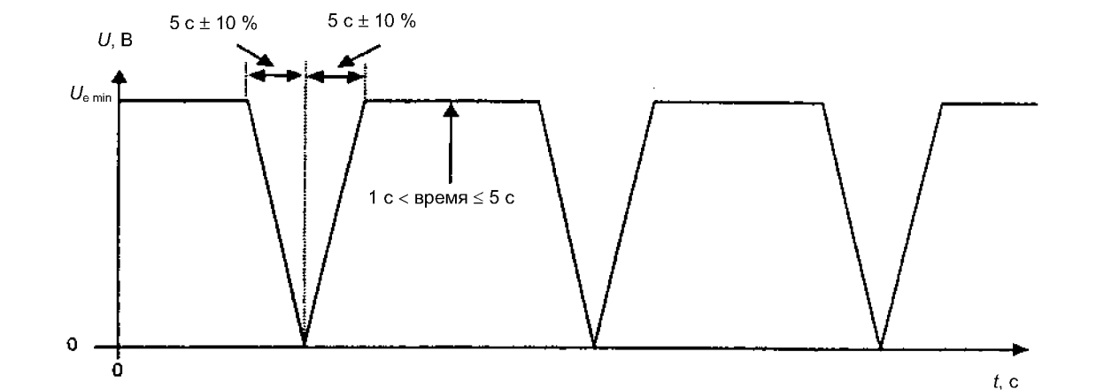
Рисунок 9 – Испытание на быстрое изменение напряжения питания
