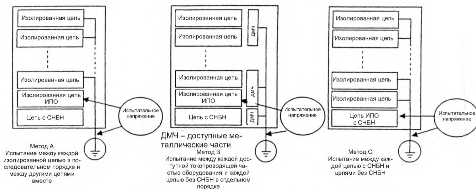
Рисунок 13 – Методы испытания на электрическую прочность диэлектрика
