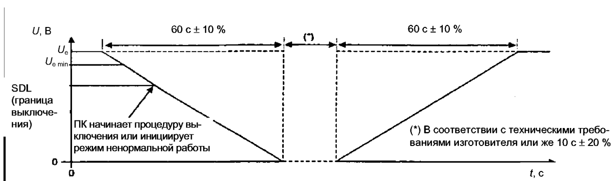
Рисунок 8 – Испытание на устойчивость функционирования при постепенной остановке/постепенном запуске
