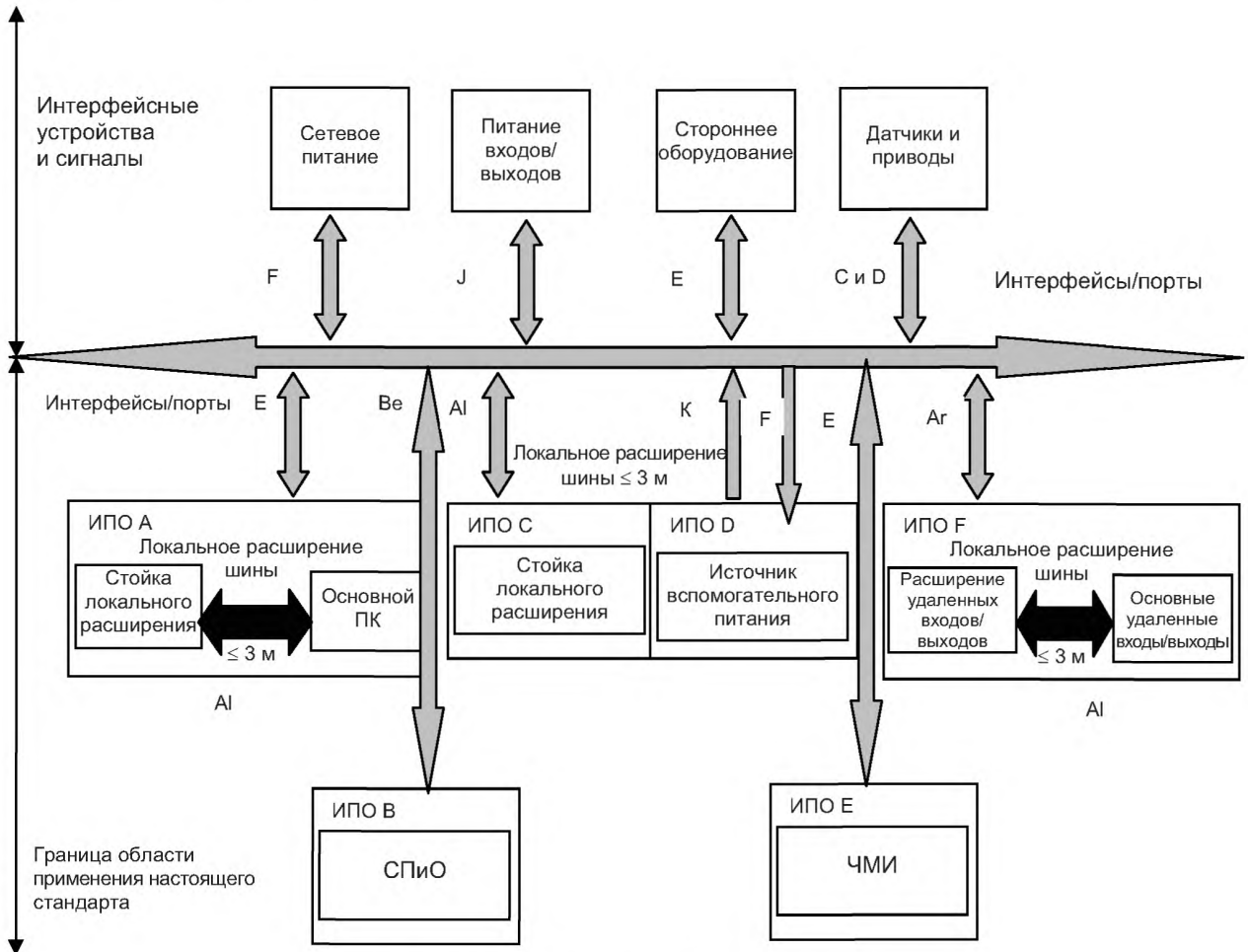
Рисунок 1 – Конфигурации испытываемого оборудования
