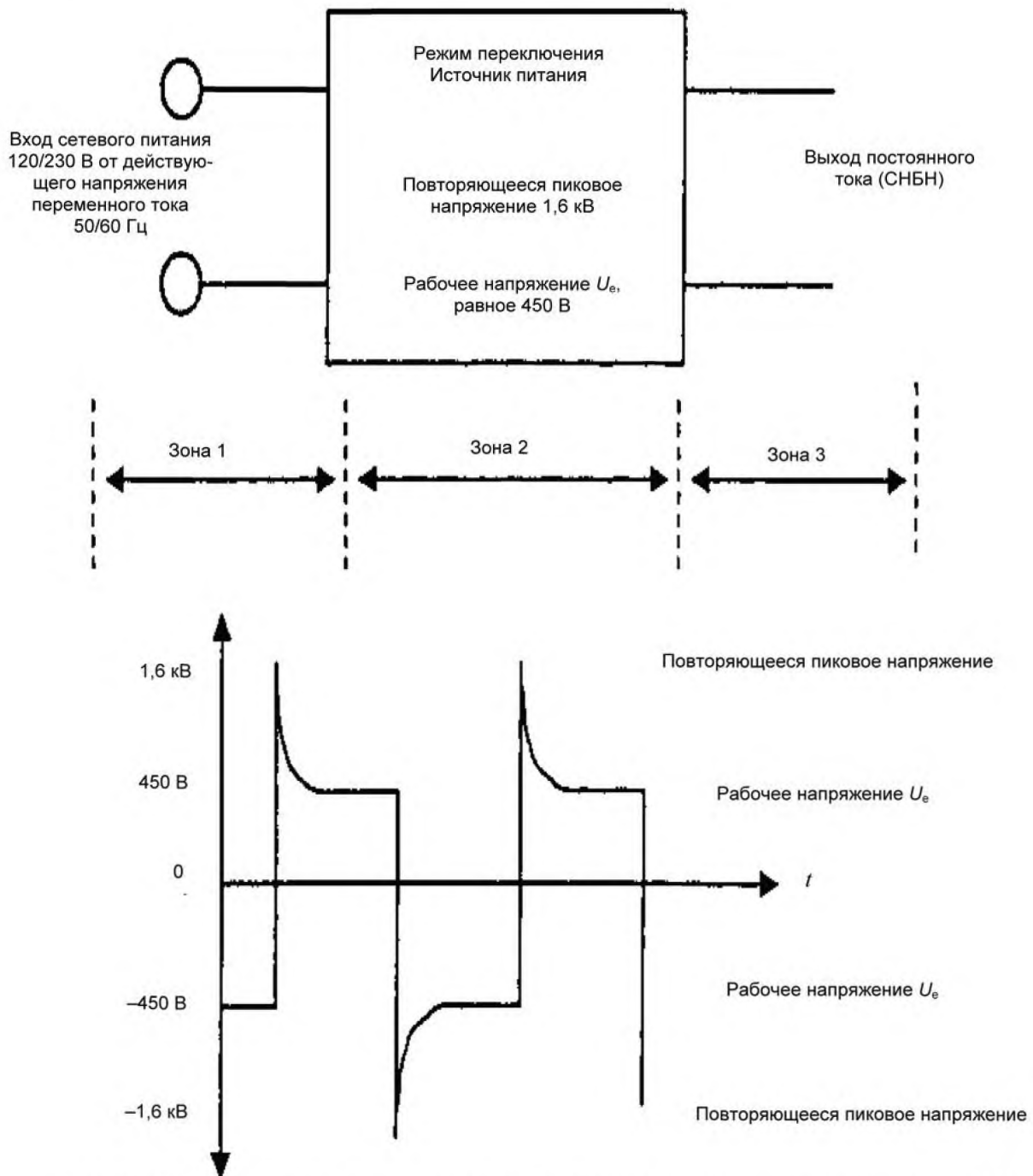
Рисунок Е.1 – Длина пути утечки для цепей, в которых создаются повторяющиеся пиковые напряжения
