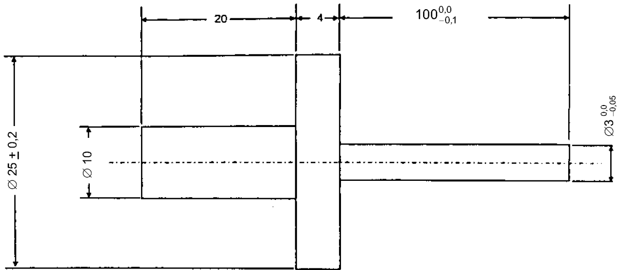
Рисунок С.4 – Испытательный штифт 100 × 3 мм
