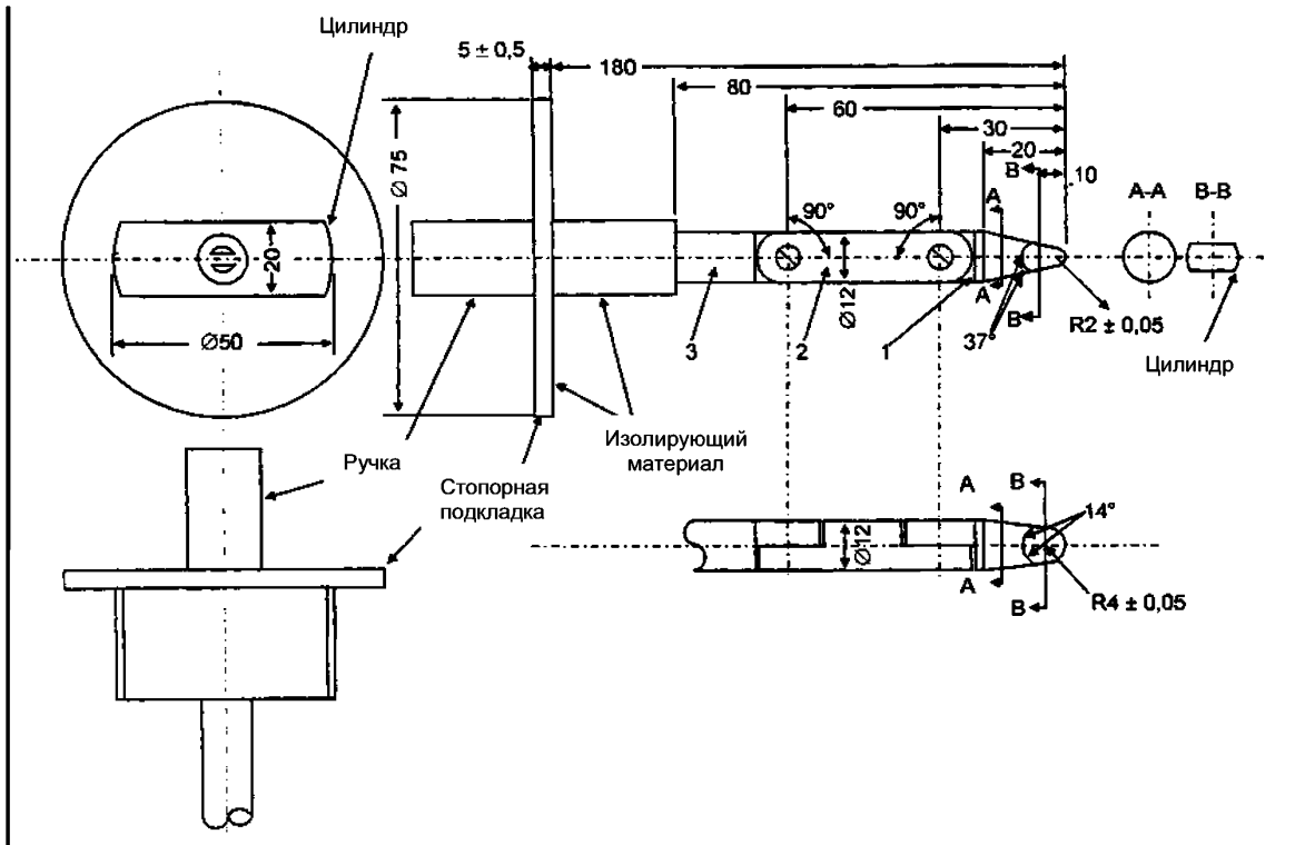
Рисунок С.1 – Шарнирный испытательный палец
