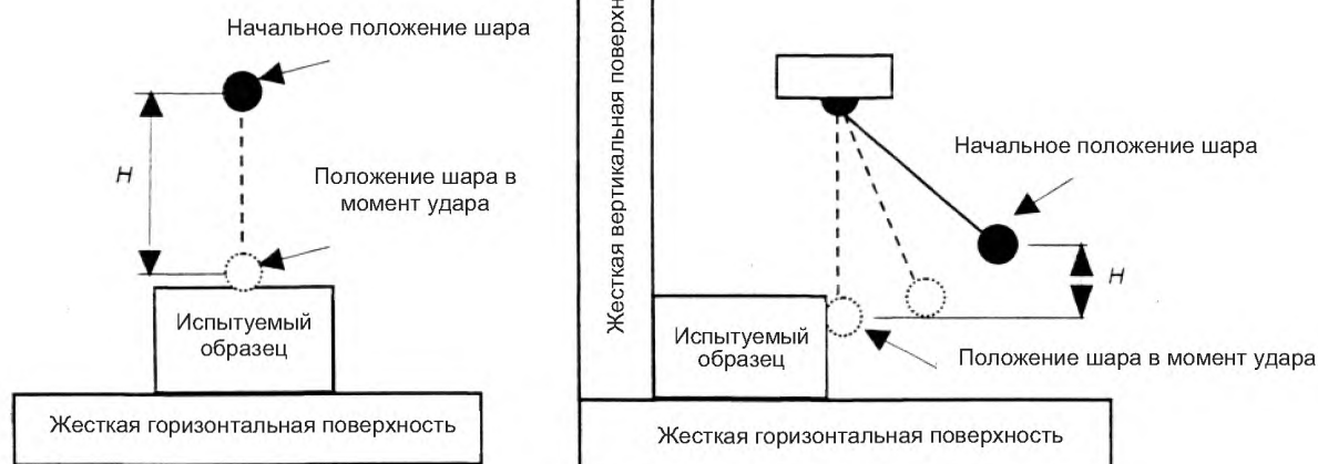
Рисунок 12 – Метод испытаний на ударостойкость
