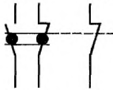
Рисунок L.1 – Пример схемы механически связанных замыкающего и размыкающего контактов и несвязанного размыкающего контакта
