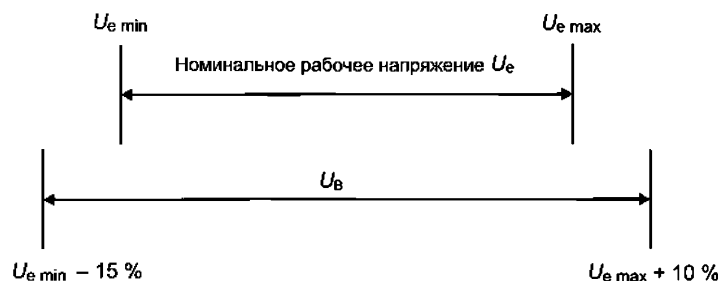
Рисунок Н.1 – Соотношение между U_e и U_B
