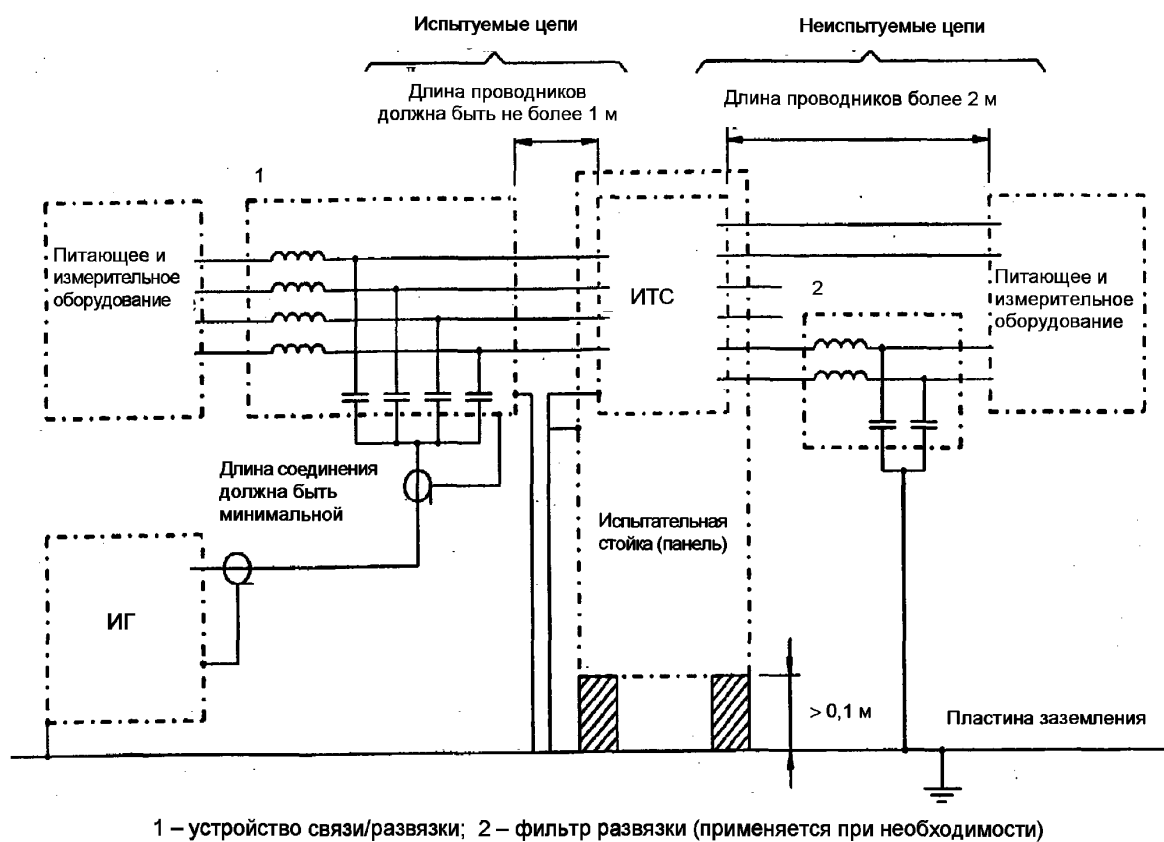
Рисунок 1 – Пример рабочего места для испытаний с применением устройства связи/развязки
