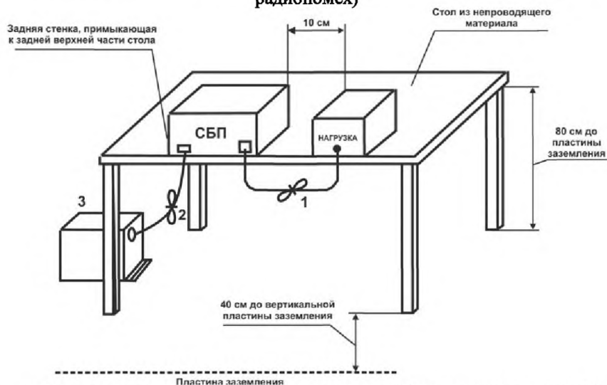
Рисунок 3 — Рабочее место для испытаний настольных СБП (измерение напряжения радиопомех)
