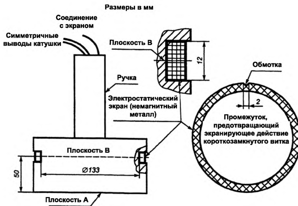
Рисунок А.1 – Конструкция рамочного датчика
