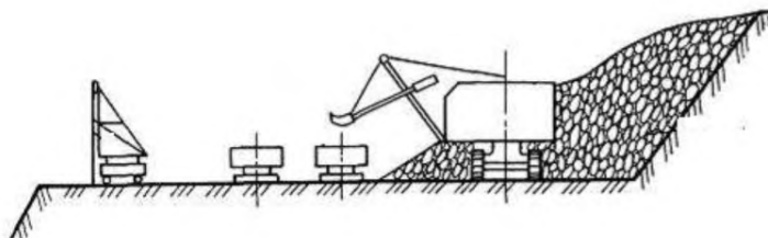
Рисунок 2.3 — Совмещение работ на уступе
