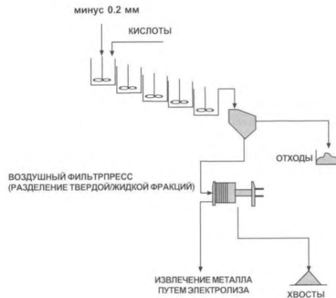
Рисунок 2.27 — Схема выщелачивания перемешиванием
