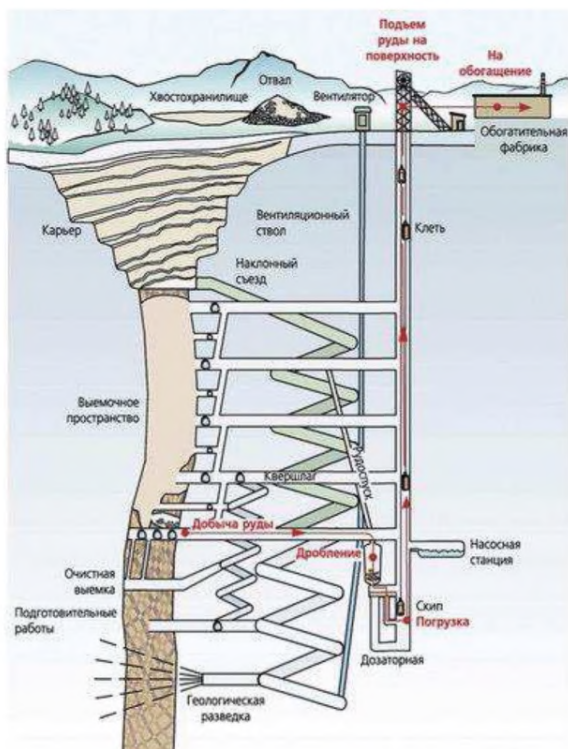
Рисунок 2.6 — Схема вскрытия месторождения
