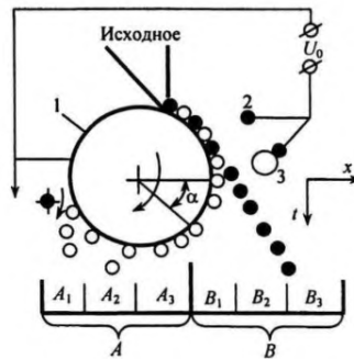
Рисунок 2.34 — Барабанный электрический сепаратор
