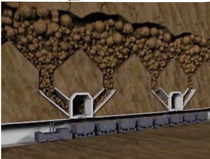
Рисунок 2.12 — Выпуск руды из блока
