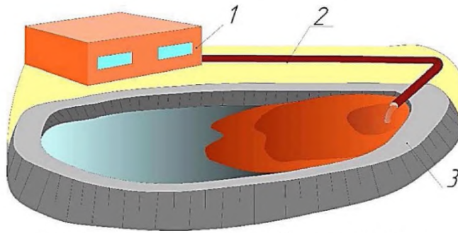
1 — обогатительная фабрика; 2 — пульпопровод; 3 — дамба наливного хвостохранилища
