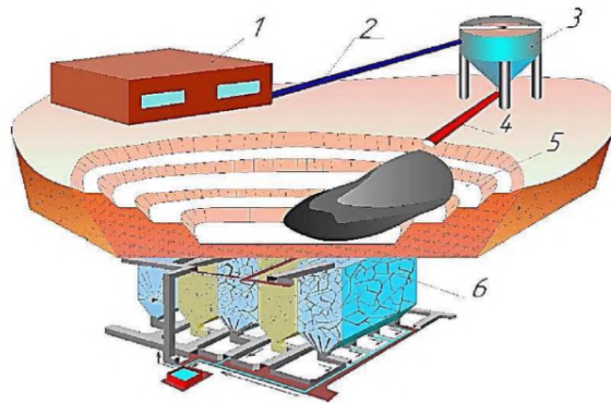
1 — обогатительная фабрика; 2 — пульпопровод; 3 — пастовый сгуститель; 4 — выработанное пространство карьера; 5 — подземные горные выработки; 6 — искусственный массив (перемычка).
