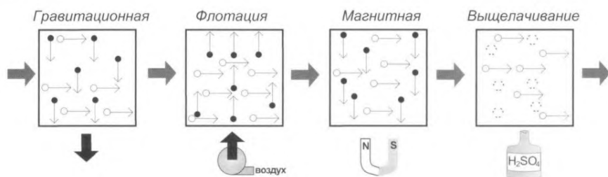
Рисунок 2.24 — Основные методы обогащения
