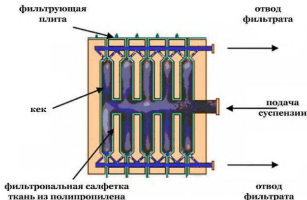
Рисунок 2.36 — Принципиальная схема фильтровальной камеры пресс-фильтра
