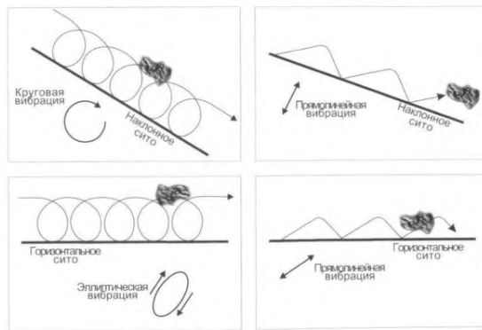
Рисунок 2.23 — Движение просеивающей среды
