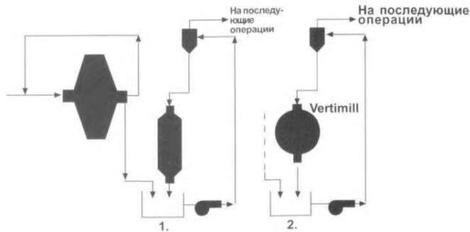
Рисунок 2.21 — Типовая схема измельчения: мельница полсамоизмельчения + шаровая мельница + мельница типа VertiMill
