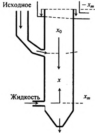
Рисунок 2.29 — Гравитационно-классифицирующий столбик
