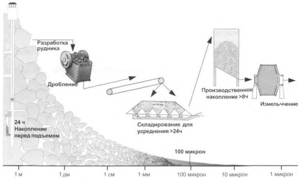
Рисунок 2.16 — Накопление руд
