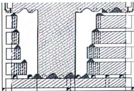
Рисунок 2.8 — Камерная система с отбойкой из поэтажей и закладкой твердеющими смесями
