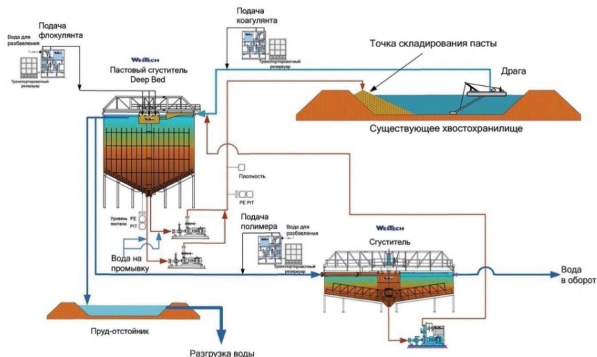
Рисунок 2.38 — Принципиальная схема пастового сгущения хвостов
