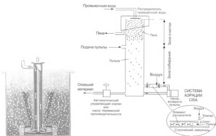
Рисунок 2.35 — Флотационные ячейки чанового и колонного типа
