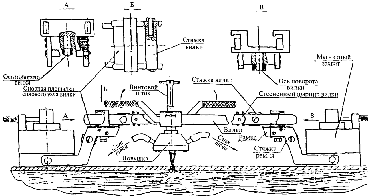
Рис. П-3.17. Схема устройства «Мост-вилка» с рычажно-винтовым управлением процессом герметизации
