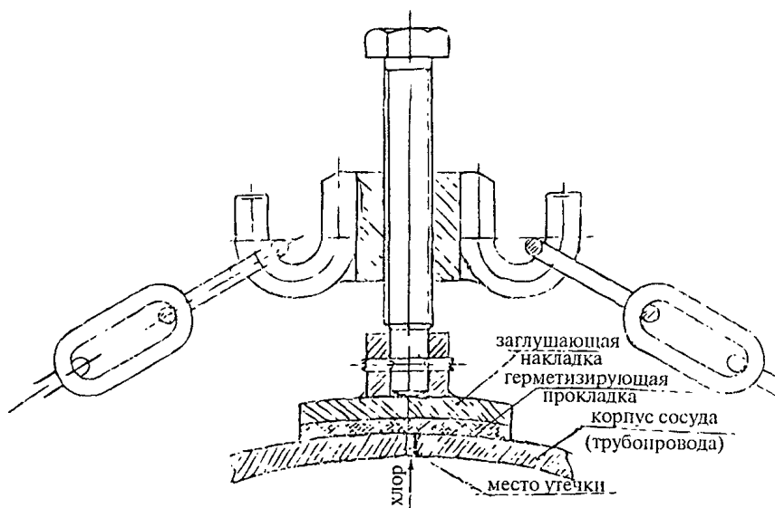
Рис. П-2.1. Устройство для устранения утечек хлора
