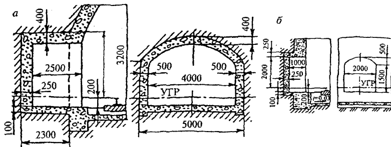
Рис. 15. Камеры и ниши в железнодорожных тоннелях
