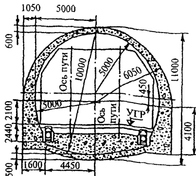
Рис. 14.2. Двухпутный тоннель с обратным сводом
