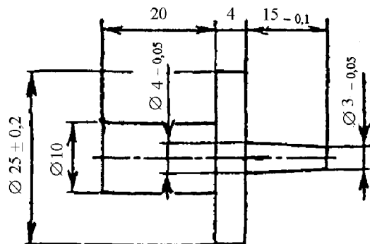
Рисунок 2 – Испытательный щуп
