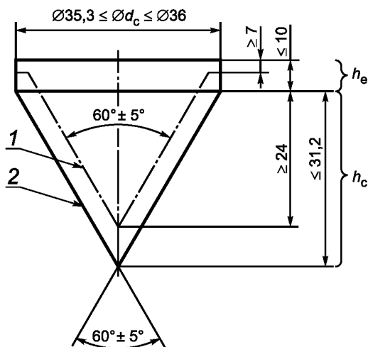
Рисунок 4 — Требования к допускам при применении наконечника с A_c = 1000 \text{ мм}^2
