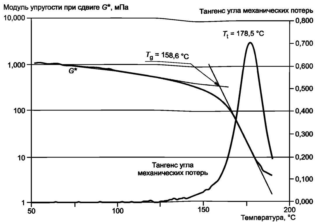
Рисунок 8 — Динамические методы определения температуры стеклования T_g после отверждения или T_t линейным изменением температуры
