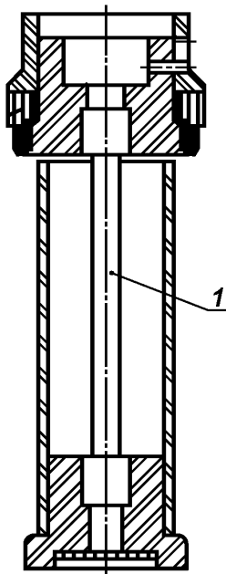
1 — шток с торсионной пружиной
