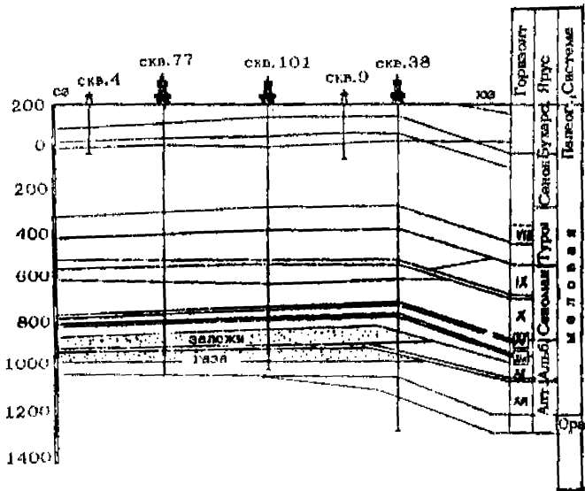
Геологический профиль проходящий через скважины 4, 77, 101, 9, 38
