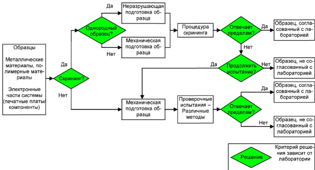
Рисунок 1 — Блок-схема проведения испытаний
