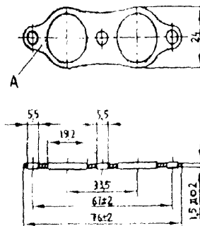
Рисунок 5 – Пластина для крепления колец
