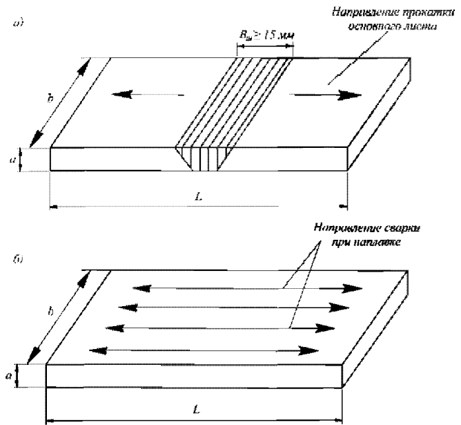
Рис. 4.8.4.3.2 Образцы для испытаний на стойкость против межкристаллитной коррозии: а — металла шва в составе сварного соединения; б — наплавленного металла плакирующего слоя
