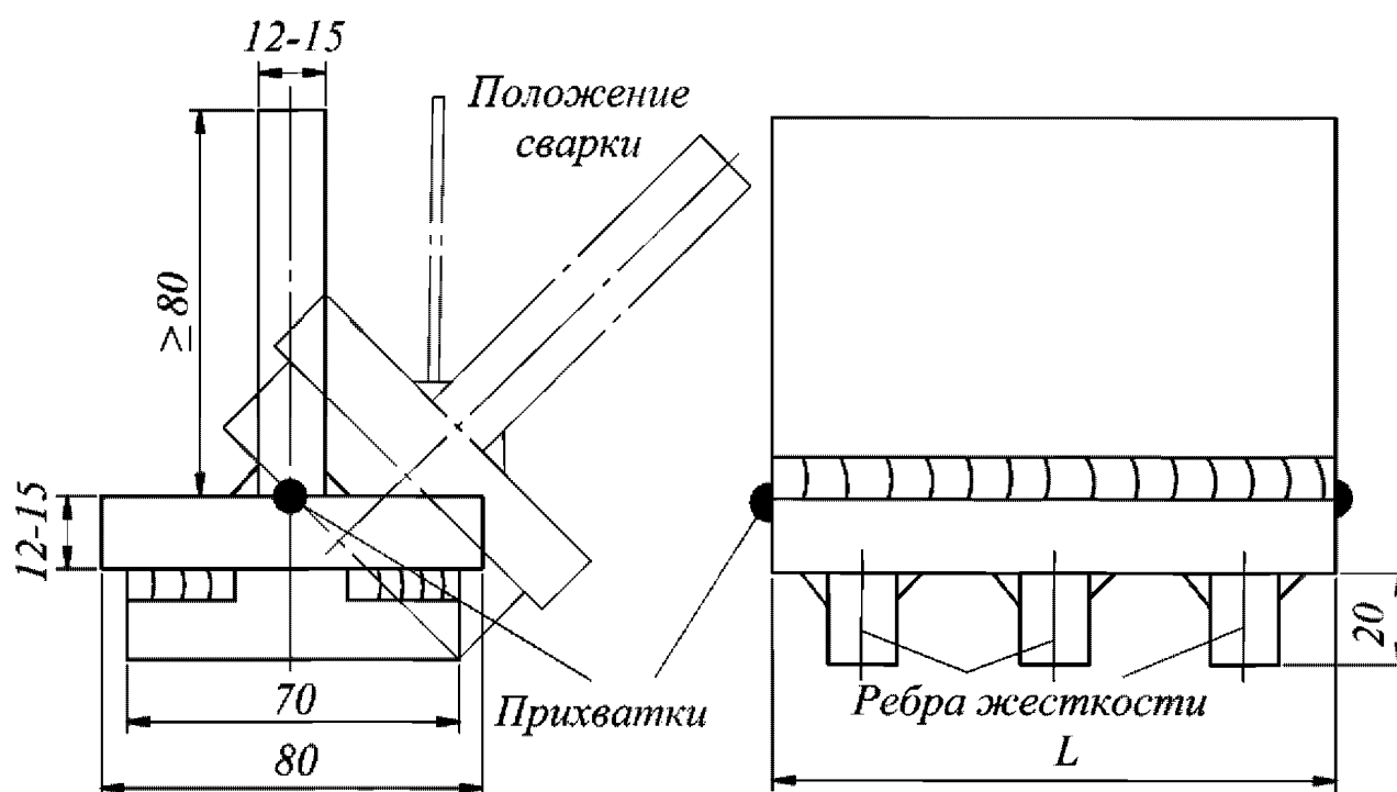
Рис. 4.2.4.1 Тавровая проба для оценки стойкости сварных соединений к образованию горячих трещин: L = 120 мм для ручной сварки покрытыми электродами; L = 250 мм для полуавтоматической сварки плавящимся электродом; L = 200 мм для ручной сварки неплавящимся электродом в среде инертного газа
