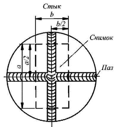
Рис. 3.1.5.11-1: a — длина снимка, равная ~500 мм; b — ширина снимка, равная ~100 мм
