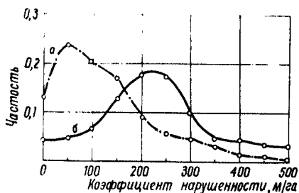
Рис.2.6. Кривые распределения тектонически нарушенных участков, соразмерных с выемочными полями лав в целом по Прокопьевско-Киселевскому месторождению: а-восточные крылья синклиналей, б-западные крылья синклиналей
