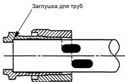
Рисунок 4 — Установка концевого фитинга на трубу
