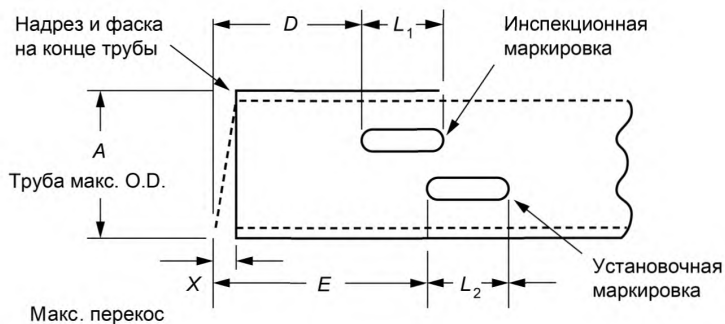
Рисунок 1 — Маркировка труб
