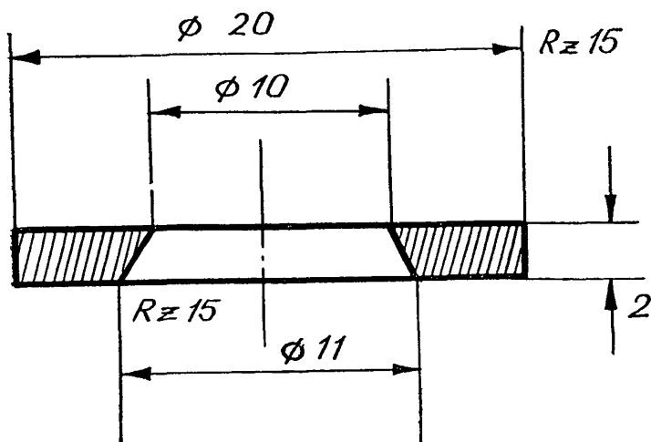
Рис. 2. Эскиз матрицы
