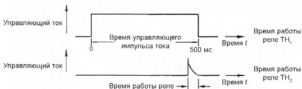
Рисунок G.2 – Подходящая цепь для формирования и приложения импульсов продолжительной длительности
