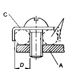
Контактные зажимы с крепежной головкой
