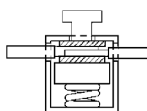
Рисунок 18 – Примеры безвинтовых контактных зажимов пружинного типа
