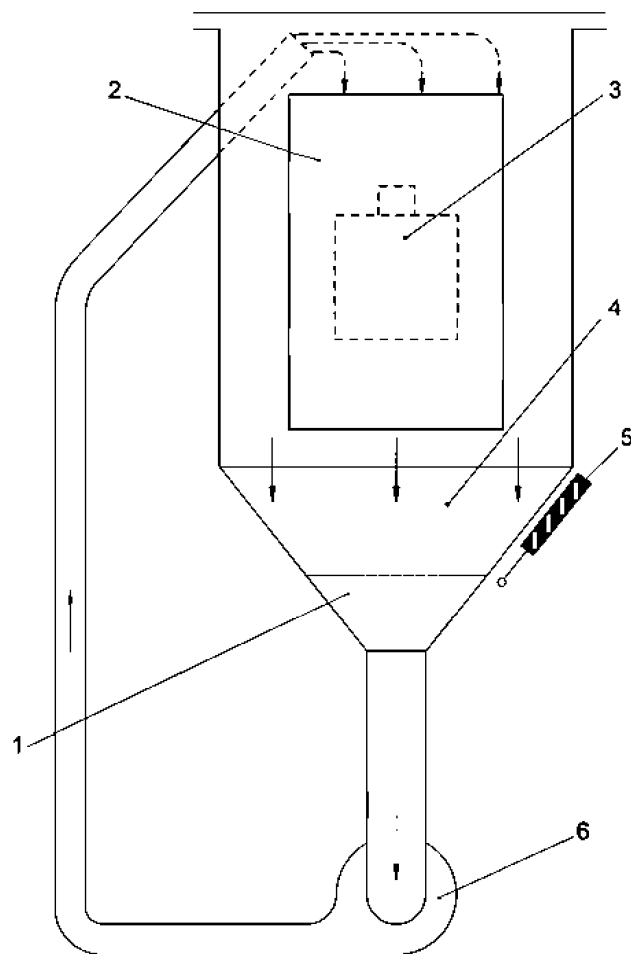
1 – проволочное сито; 2 – стеклянное окно; 3 – испытуемый светильник; 4 – поток пудры талька; 5 – вибратор; 6 – циркуляционный насос
