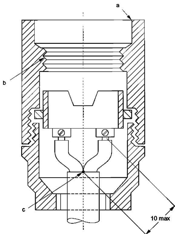
a, b, c – месторасположение термопар
