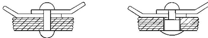
Рисунок 17 – Конструкция неразъемных соединений
