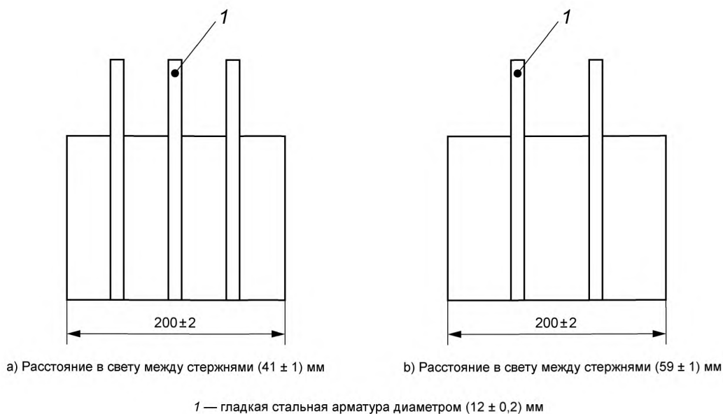
Рисунок 2 — Положение стержней в L-образной коробке
