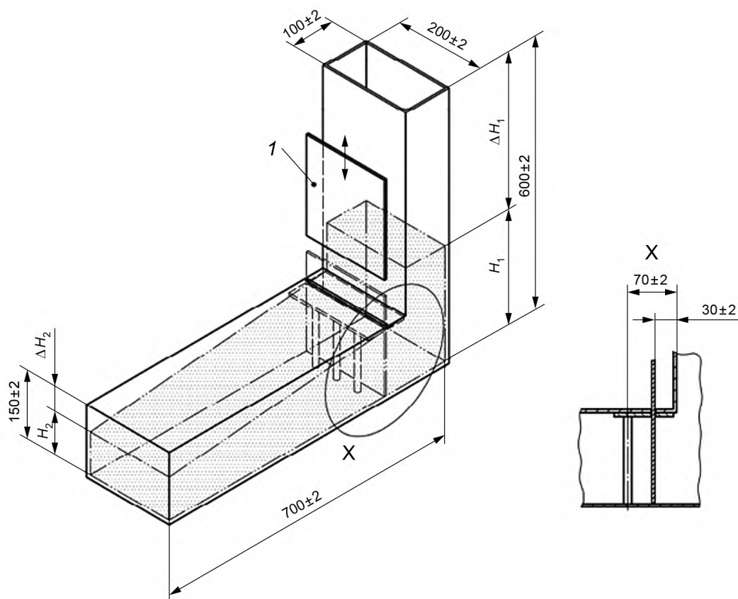
Рисунок 1 — Типовая конструкция L-образного короба с предусмотренными размерами
