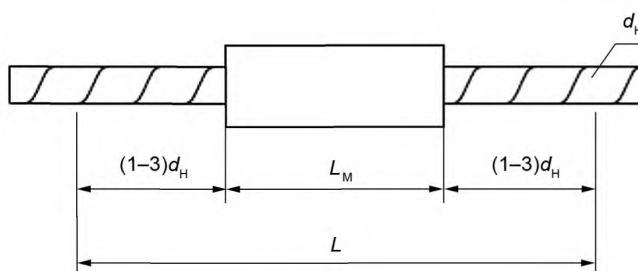
Рисунок 2 — База измерения деформаций
