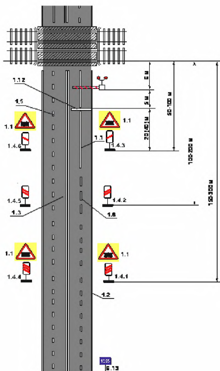
Рисунок Г.26, лист 2
