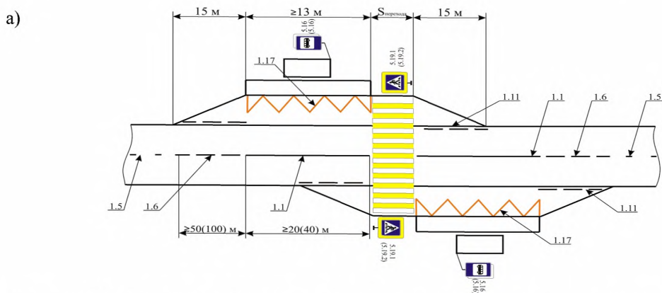
Рисунок Г.8 – Примеры применения элементов обустройства в зоне остановочного пункта маршрутных транспортных средств с заездным карманом, лист 1
