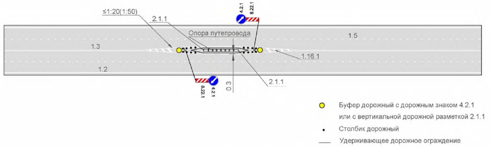
Рисунок Г.24, лист 2
