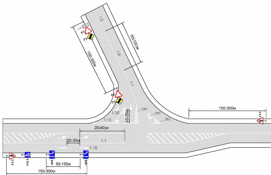
Рисунок Г.4 – Пример применения элементов обустройства на Т-образном перекрестке, лист 1
