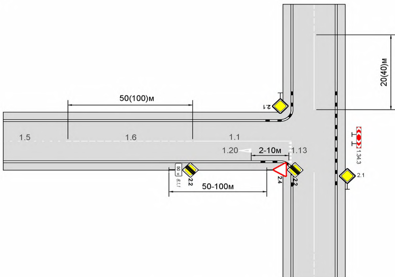
Рисунок Г.4, лист 2
