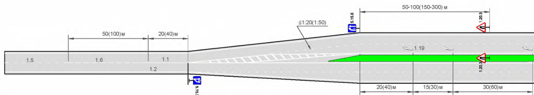
Рисунок Г.25, лист 2
