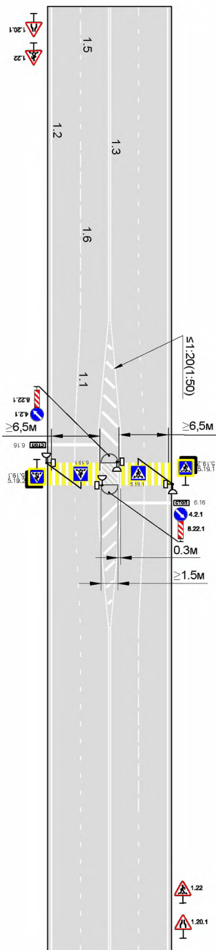
Рисунок Г.13 – Пример применения элементов обустройства при обустройстве нерегулируемого пешеходного перехода с островком безопасности
