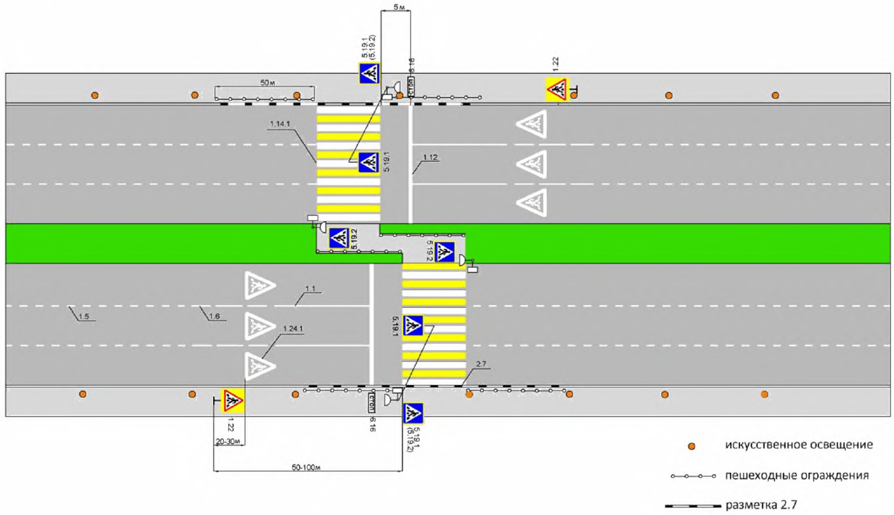
Рисунок Г.17, лист 2
