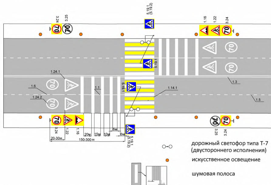
Рисунок Г.10 – Пример применения элементов обустройства при обустройстве нерегулируемого пешеходного перехода вне населенного пункта
