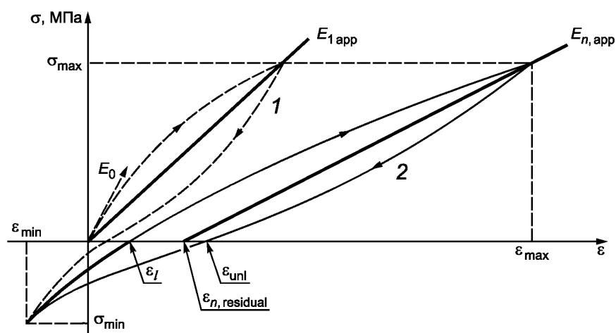
Рисунок 3 — Знакопеременный цикл нагружения
