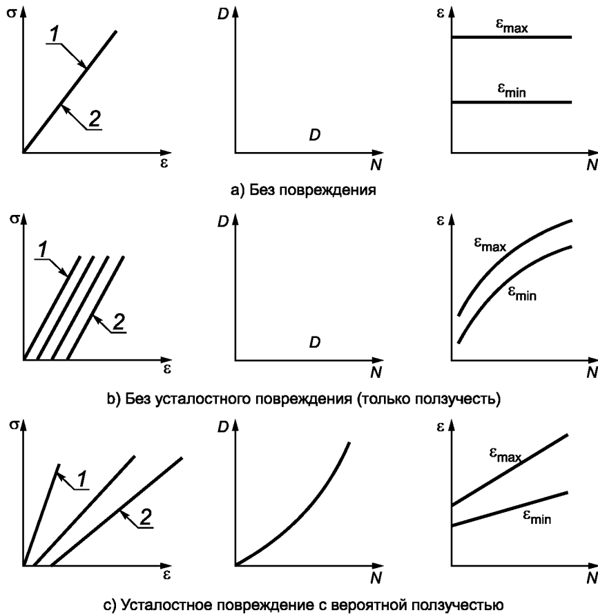
Рисунок А.1 — Схематическое развитие E: а) без повреждения, б) ползучесть, без усталостного повреждения, и с) усталостное повреждение с вероятной ползучестью
