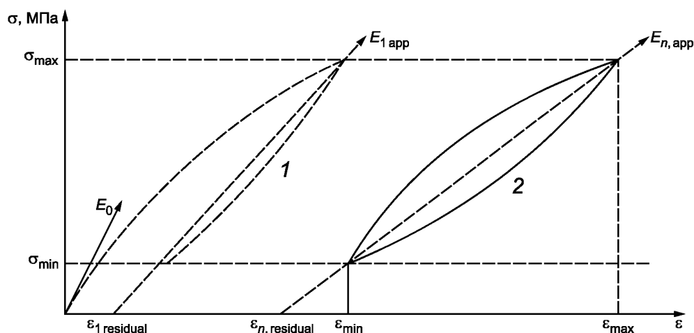
Рисунок 4 — Знакопостоянный цикл нагружения
