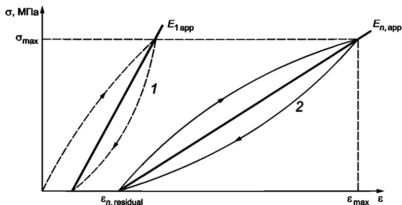
Рисунок 2 — Отнулевой цикл нагружения
