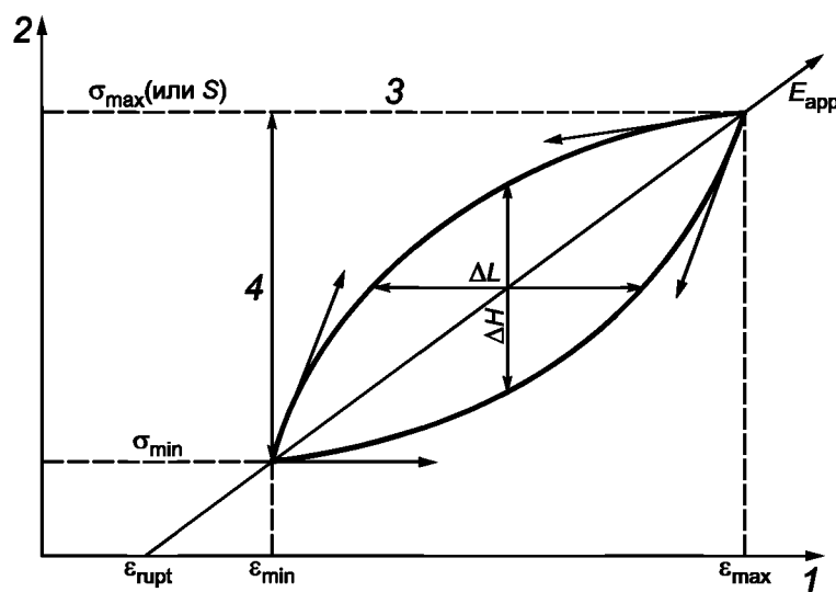
Рисунок 2 — Параметры для оценки усталостной долговечности
