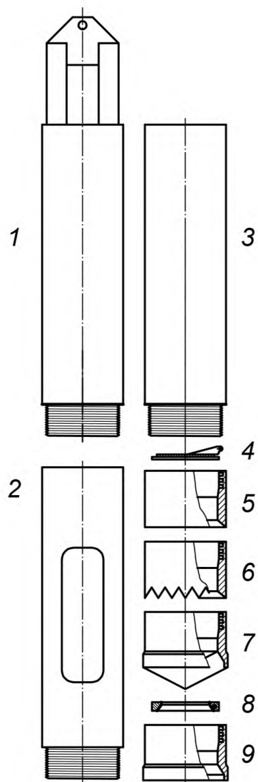
1 — подвесная секция; 2 — секция с окном; 3 — гладкая секция; 4 — откидной клапан; 5 — гладкий башмак; 6 — зубчатый башмак; 7 — башмак, заканчивающийся зубилом; 8 — кольцо бура для мягких пород; 9 — башмак бура для мягких пород
