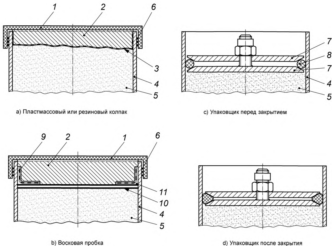
1 — пластмассовый или резиновый колпак; 2 — грунт для заполнения пространства между верхом трубки и пробой; 3 — пластиковое полотно; 4 — трубка с пробой; 5 — проба; 6 — герметизирующие выступы; 7 — металлическая пластина; 8 — резиновое уплотнение; 9 — липкая лента; 10 — два слоя плавленного воска; 11 — восковая пробка
