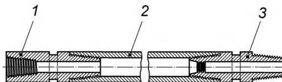
1 — муфта бурового замка; 2 — труба штанги; 3 — ниппель бурового замка
