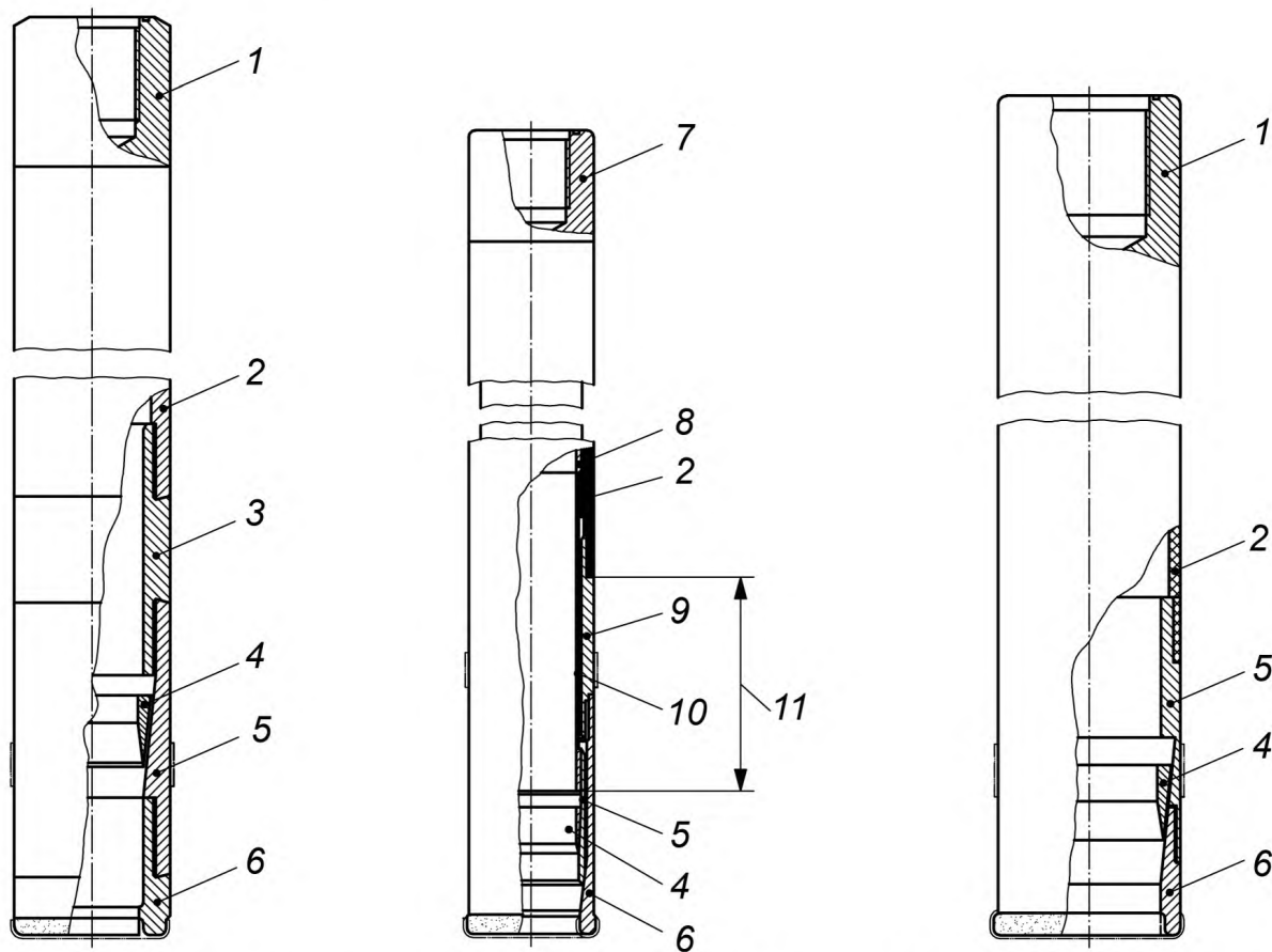
а) Колонковая труба типа Z — сборка
