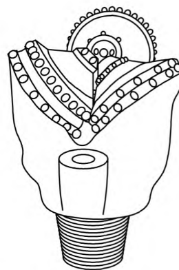
Рисунок С.12 — Долото со вставными зубьями из карбида вольфрама
