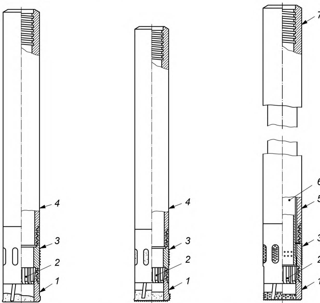
а) Одиная колонковая труба проекта WG — сборка а
