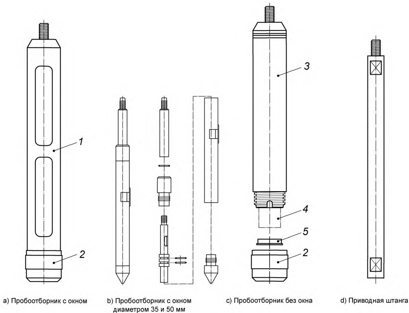
1 — окно в трубе устройства для отбора проб; 2 — башмак; 3 — труба устройства для отбора проб; 4 — пластмассовый вкладыш; 5 — держатель пробы
