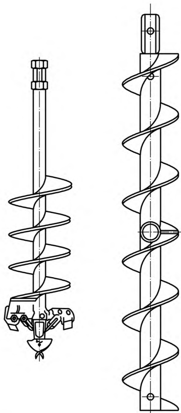
Рисунок С.27 — Непрерывный спиральный шнековый бур
