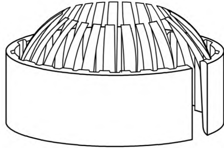
d) С прорезями изнутри и пальцами корзиночного типа
