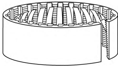
e) С прорезями, зубчатый изнутри и с пальцами корзиночного типа
