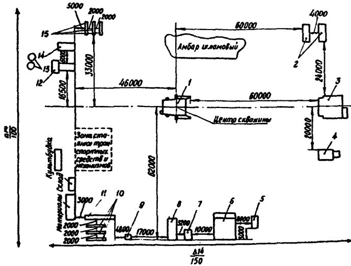
Рис. 6. Схема расположения блоков, вспомогательных узлов и оборудования буровой установки "Уралмаш-125БЭ" перед монтажом I - вышечно-лебедочный блок; 2 - емкости ЦСГО приемные; 3 - силовой блок; 4 - гидромешалка; 5 - склад химреагентов; 6 - насосный блок; 7 - электрокотельная; 8 - подстанция; 9 - инструментальная площадка; 10 - стеллажи приемного моста l = 9 м; 11 - секционный приемный мост; 12 - ЦСГО; 13 - емкость долива; 14 - емкость ЦСГО промежуточная; 15 - стеллажи приемного моста
