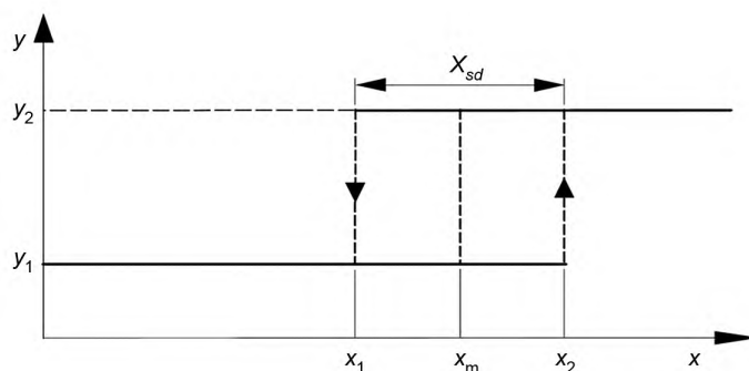
Рисунок 1 — Прибор с двумя устойчивыми состояниями
