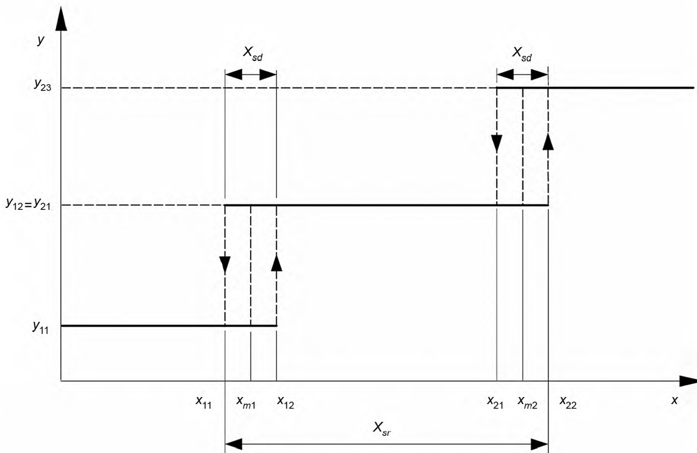
Рисунок 4 — Прибор с тремя устойчивыми состояниями
