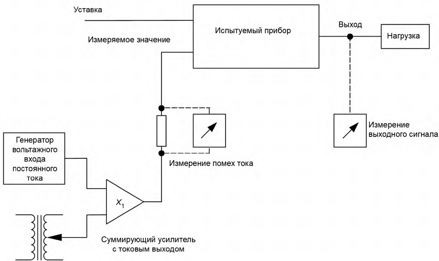
Рисунок 3b — Токвый вход
