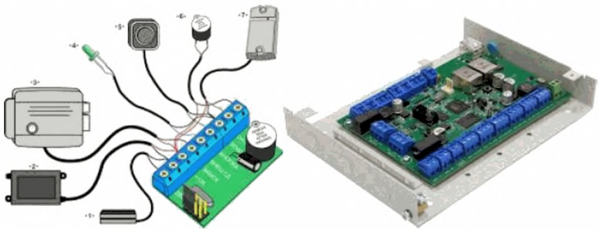
Рисунок 15. Контроллер доступа.
