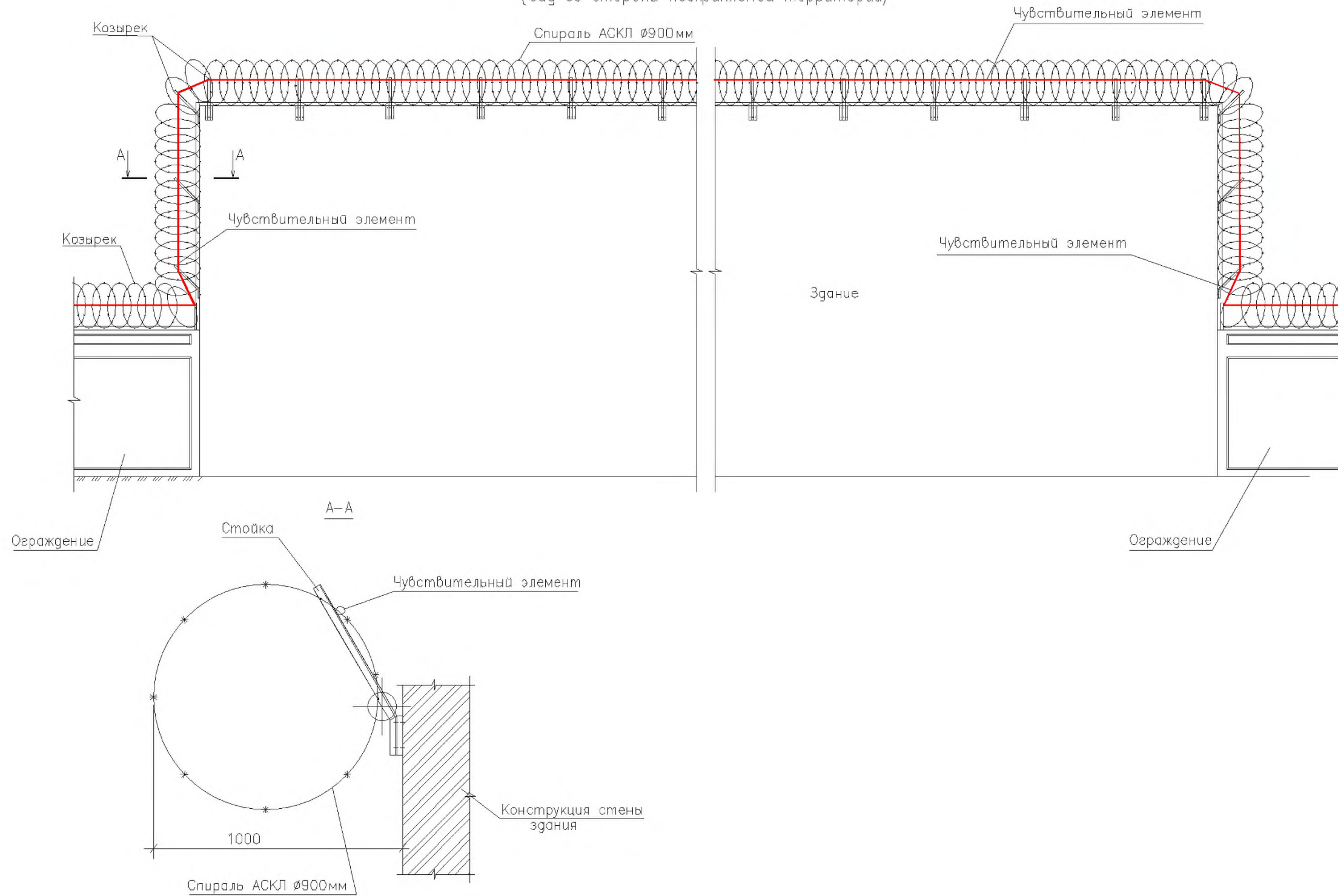
Схема блокировки от проникновения через здание вибрационным извещателем (вид со стороны не охраняемой территории)
