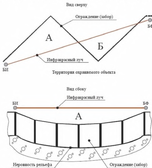
Рисунок 21. Неправильное использование активного ИК извещателя.
