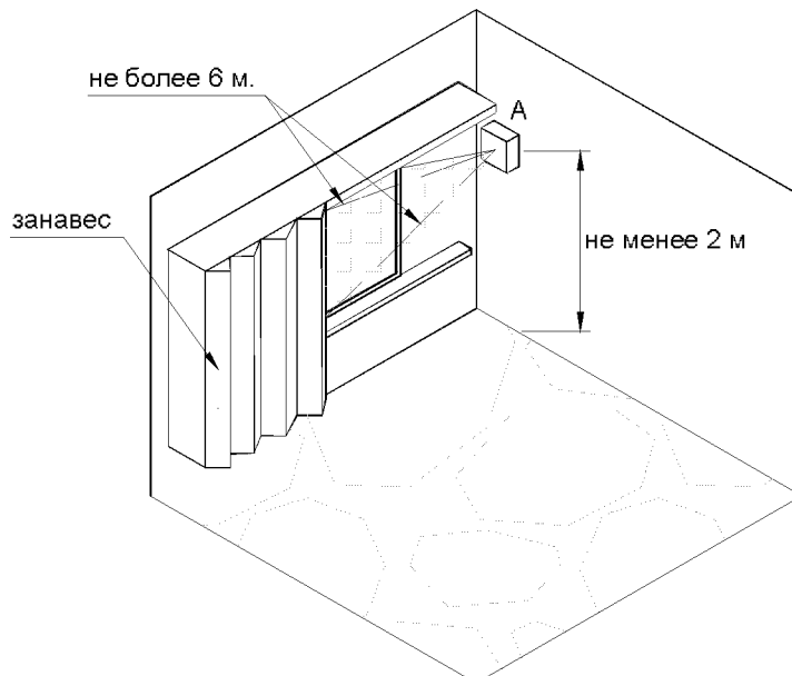
Установка извещателя между стеклом и занавесом (жалюзи)
