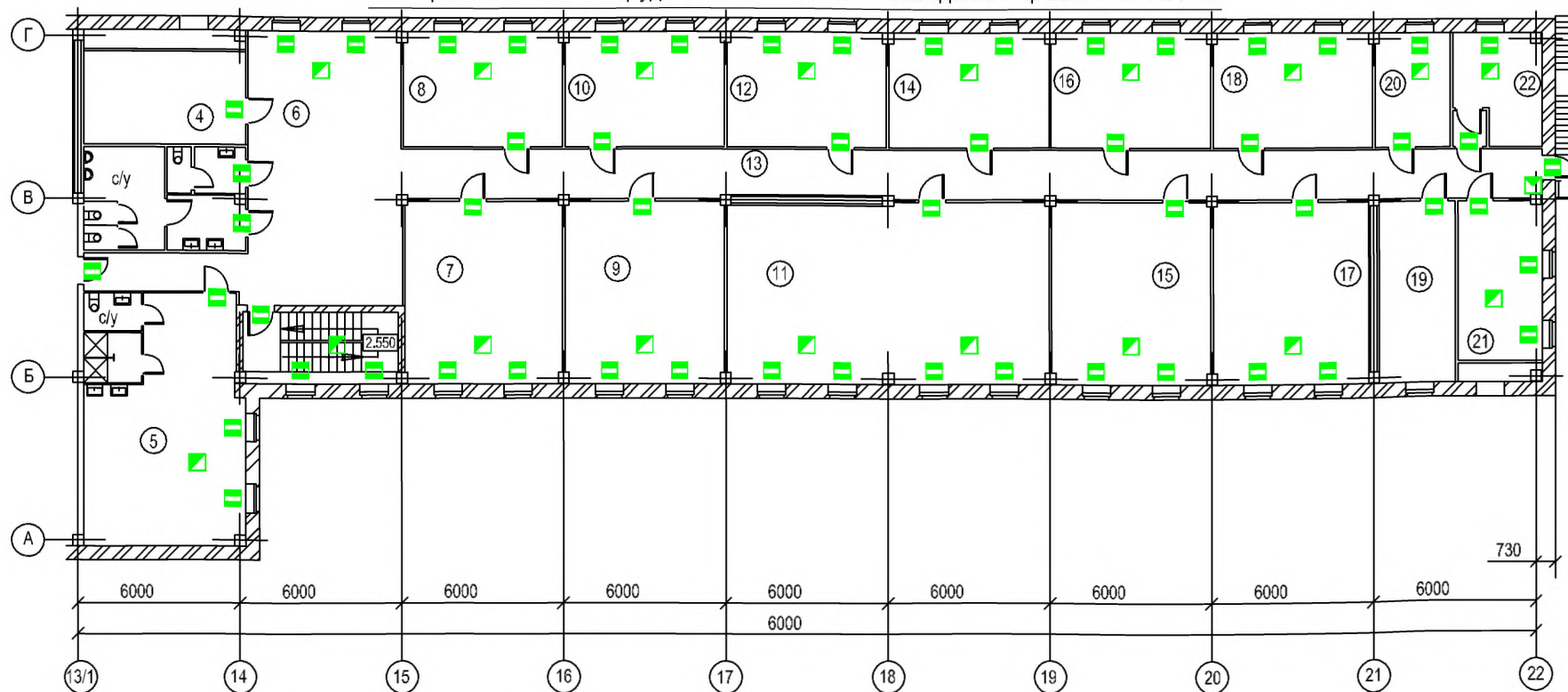
План расположения оборудования СОТС 2-го этажа здания гаража. Оси 13/1-22
