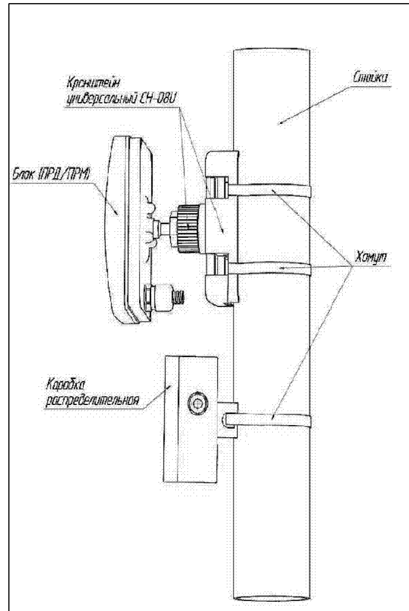
Схема монтажа извещателя охранного линейного радиоволнового
