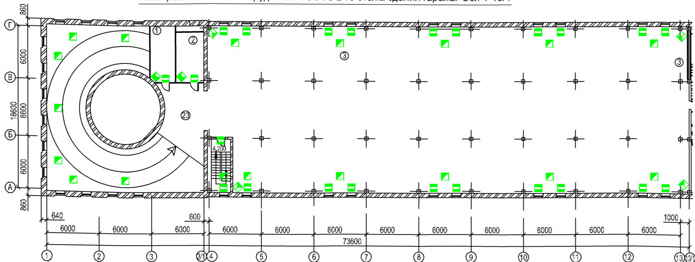
План расположения оборудования СОРТС 2-го этажа здания гаража. Оси 1-13/1
