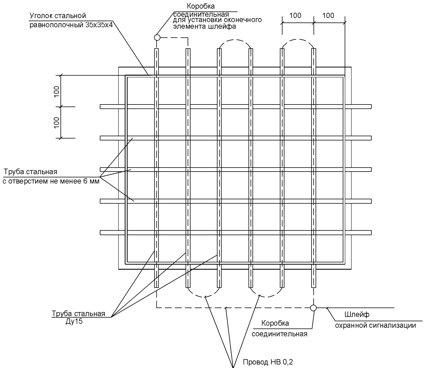
Схема блокировки окна омическим извещателем.
