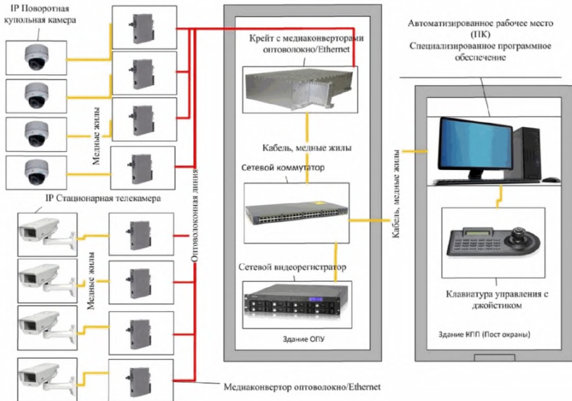
Рисунок 20. Структурная схема СОР на базе IP-видеонаблюдения.
