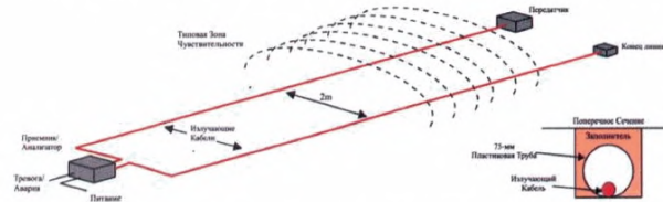
Рисунок 31. ЛВВ – извещатель.
