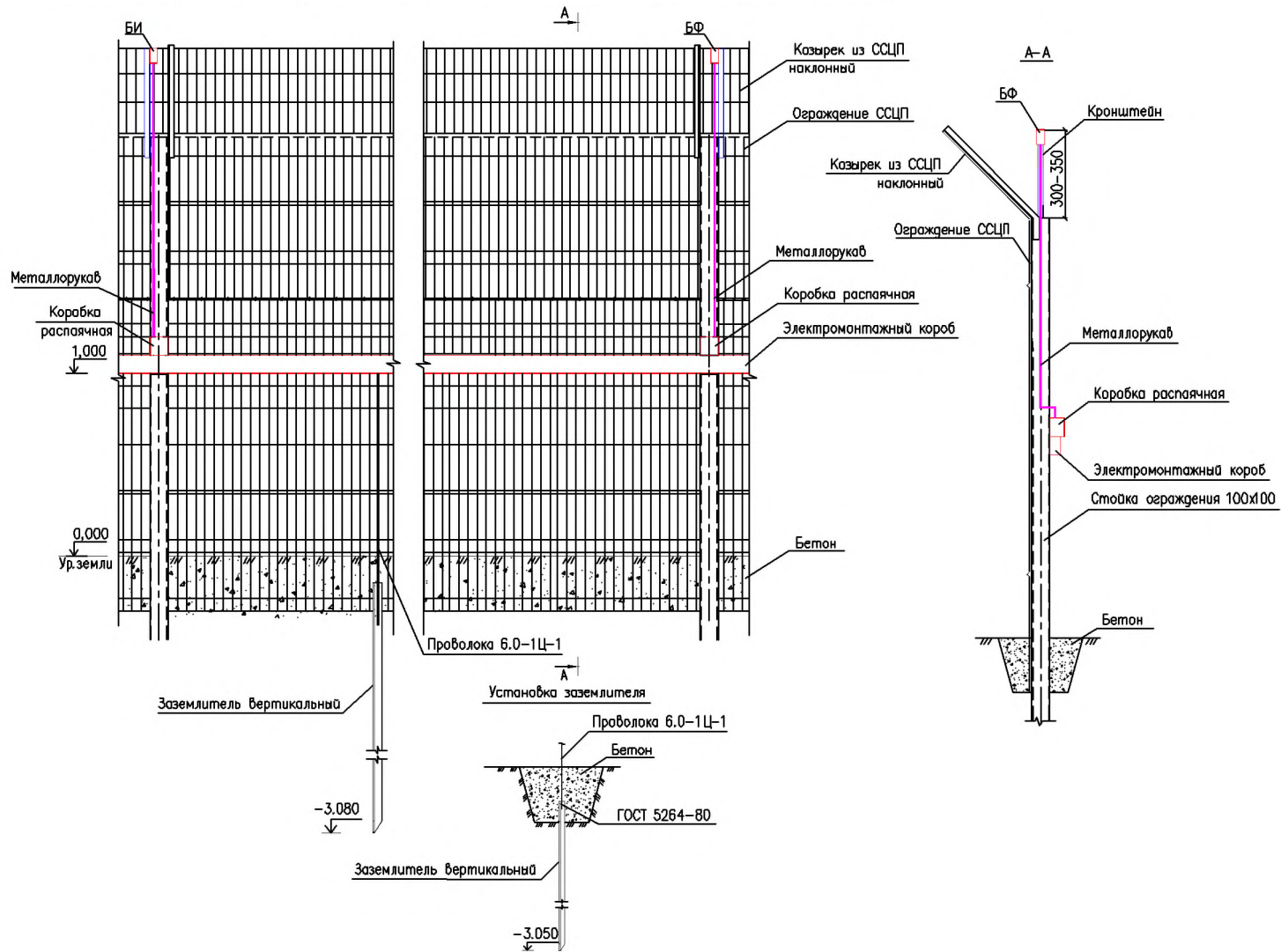
Схема блокировки ограждения от перелазу инфракрасным линейным извещателем
