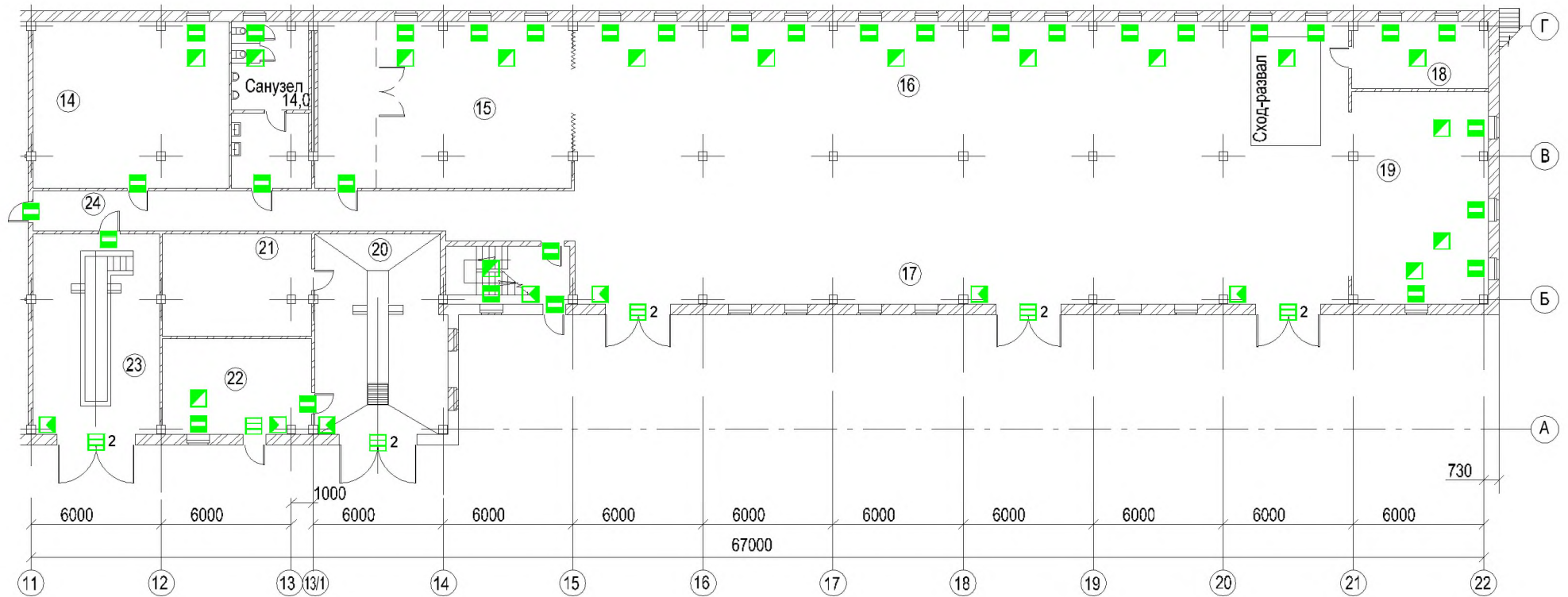
План расположения оборудования СОТС 1-го этажа здания гаража. Оси 11-22
