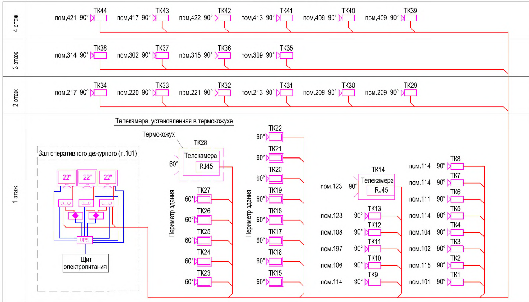
Структурная схема СОТ ЛОВД СОТ построена с использованием сетей телевизионных камер с передачей электропитания PoE.
