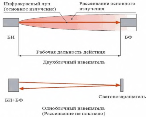
Рисунок 20. Схема активного ИК извещателя.
