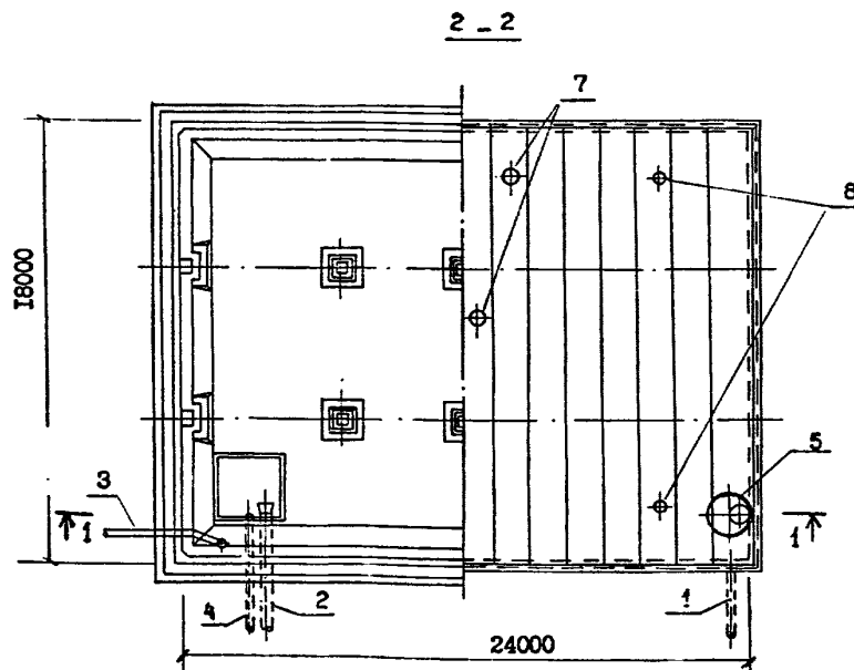
ЭКСПЛИКАЦИЯ ОБОРУДОВАНИЯ
