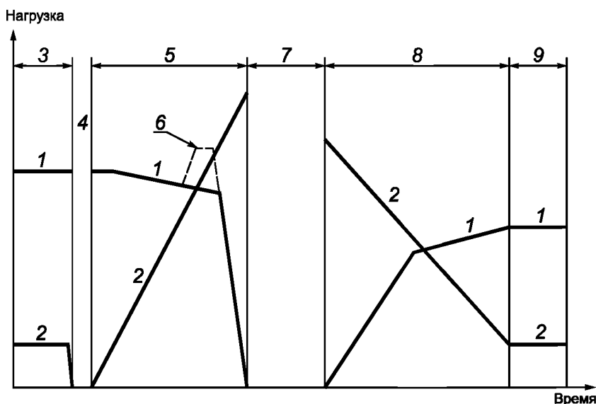
1 — нагрузка; 2 — время; 3 — «рулежка» перед взлетом; 4 — пауза 7 с в соответствующих случаях; 5 — взлет; 6 — пиковая нагрузка при отрыве носового колеса (в соответствующих случаях); 7 — период нагревания или охлаждения в полете; 8 — посадка; 9 — «рулежка» после посадки
