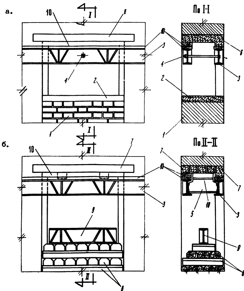
Рис.4.6. Схемы устройства домкратной ниши в оконном проеме подвала:
