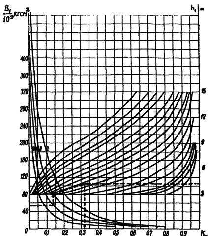
Рис. III.11. Номограмма для определения значений коэффициента взаимосвязи между горизонтальными перемещениями основания и фундамента K_x :
