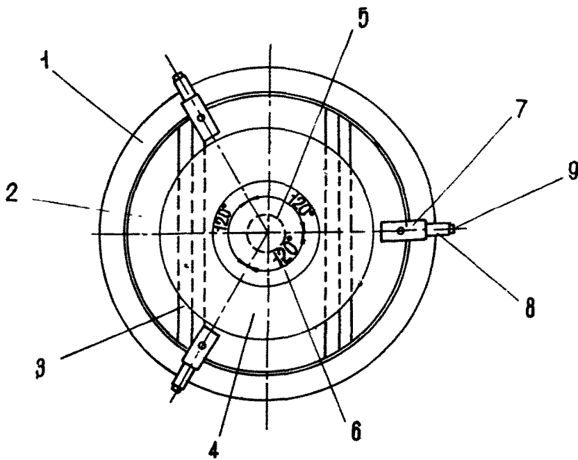
Рис. II.1. Схема испытания материала закладки на усадку: 1-стальная обѐйма; 2-стальная распределительная плита; 3-призматическая балочка; 4-распределительная балка, 5-стальной шарик; 6-загрузочная плита; 7-индикатор; 8-держатель; 9-крепежный винт; 10-материал закладки.
