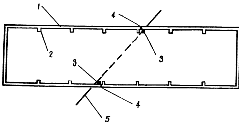
Рис.5.3. Схема разрезки на отсеки каменного бескаркасного здания с легким покрытием, расположенного под значительным углом к простиранию плитов:
