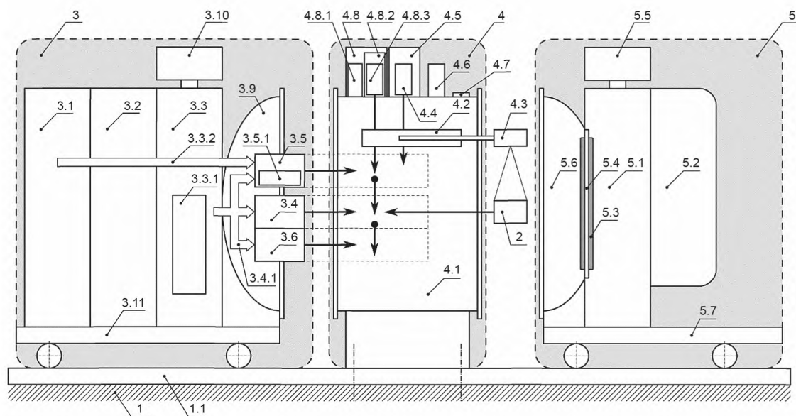
Рисунок 1 — Функциональная схема оборудования ВИПС (позиции обозначения — в соответствии с таблицей 1)
