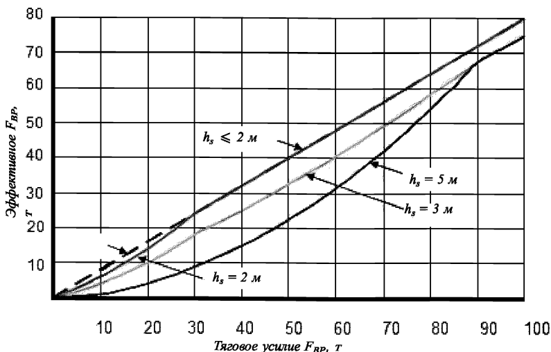
Рис. 4.5.4 Эффективное F_{BP} при различном состоянии моря (высоте волн) Примечание. Для пересчета из тонн в кН умножить на 9,8.
