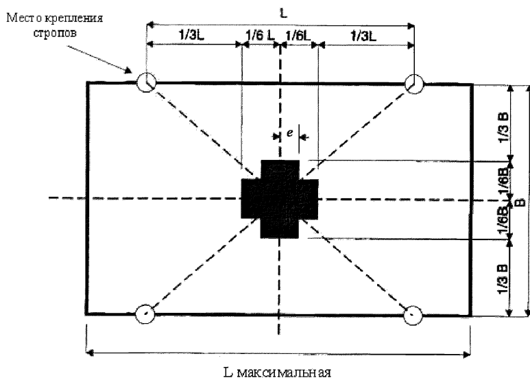
Рис. 3.3.4 Допускаемое положение ЦТ
