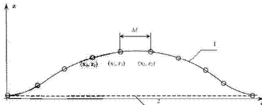
Рис. 1: 1 — фактическая трасса МПТ, 2 — первоначальная (проектная) трасса МПТ
