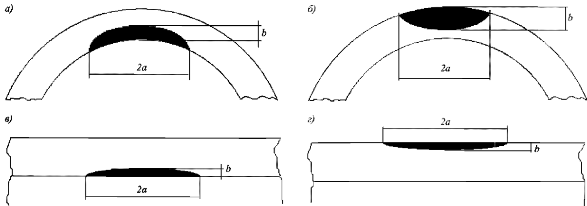
Рис. 1-1 Классификация поверхностных трещин: а) — внутренняя поперечная; б) — внешняя поперечная; в) — внутренняя продольная; г) — внешняя продольная
