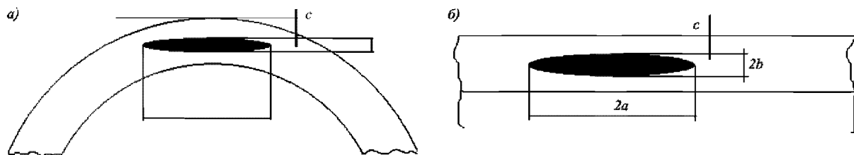
Рис. 1-2 Классификация подповерхностных трещин: а) — поперечная; б) — продольная
