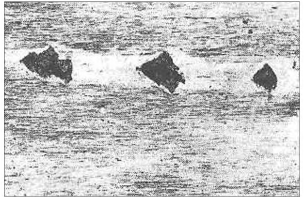
Рисунок А.13 — Закаты стали
