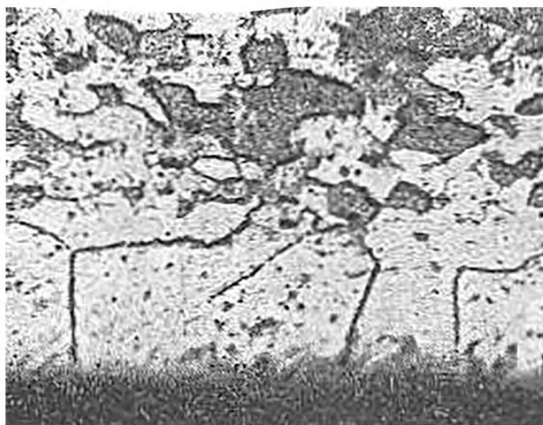
Диффузия меди в плакировку листа из сплава Д16 \times 300
