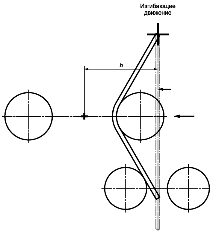
Рисунок 10 — Изгибающее движение
