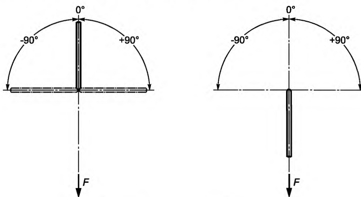
Рисунок 12 — Изгибание листов
