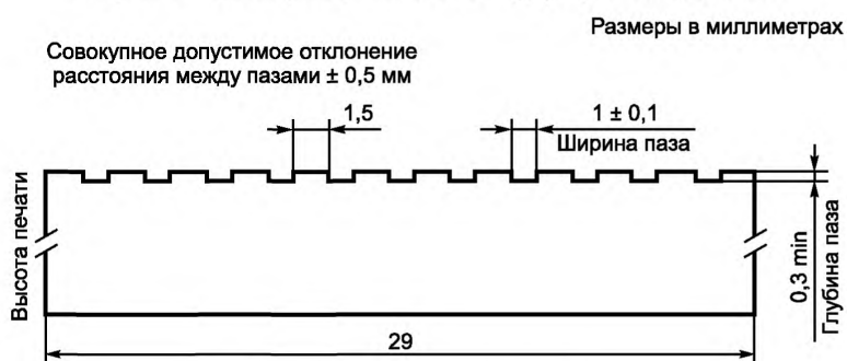
Рисунок 5 — Геометрия печати
