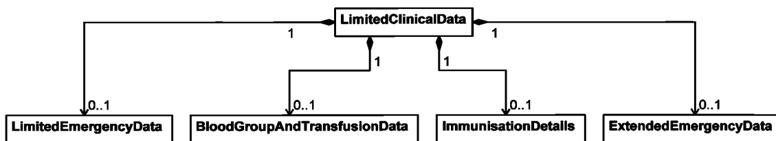
Рисунок 2 — Структура класса LimitedClinicalData
