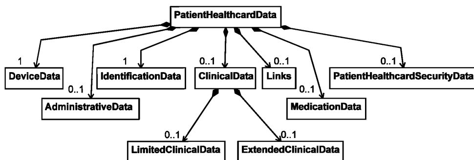
Рисунок 1 — Данные на пластиковой карте пациента. Общая структура
