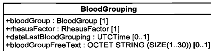
Рисунок 7 — Структура класса BloodGrouping
