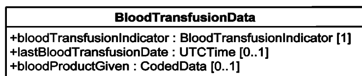
Рисунок 8 — Структура класса BloodTransfusionData
