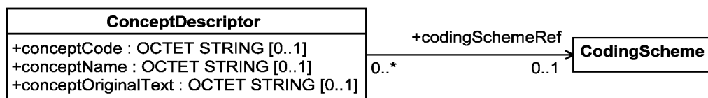
Рисунок 10 — Структура класса ConceptDescriptor
