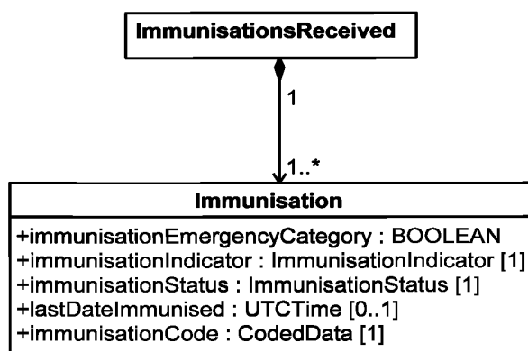
Рисунок 5 — Структура класса ImmunisationsReceived
