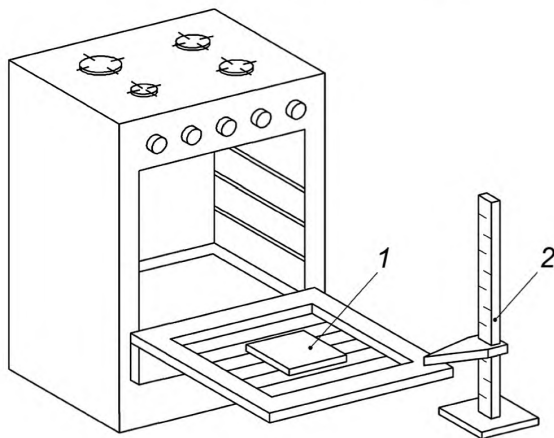
1 — испытательный груз; 2 — измерительное устройство
