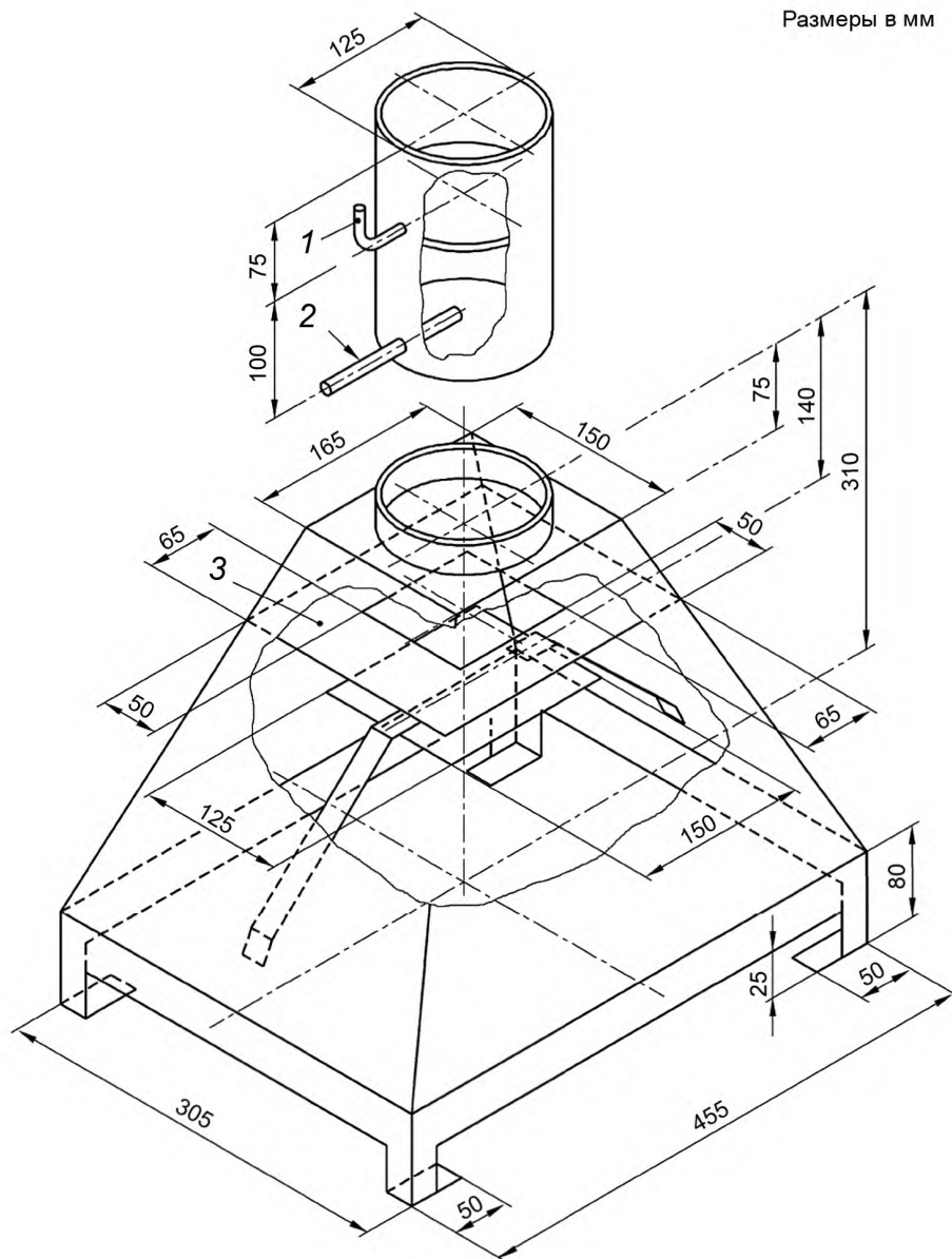
1 — поворотная заслонка; 2 — труба диаметром 8 мм; 3 — кольцеобразный диск
