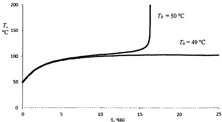
Рис. 1. Изменение максимальной температуры веществ во времени в колонне
