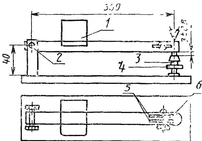
1—перемещающийся вес, 2—шарнирный палец, 3—патрон, 4—опора для патрона чтобы рычаг находился в горизонтальном положении когда усилие прилагают первый раз, 5—прорези в рычаге для более удобного зажима провода патрона, 6—отверстия для проводов
